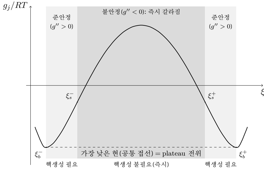
Figure 4: 가운데가 언덕이 된 자유에너지( \Omega_j = 3RT — 곡선은 식 (1.27), 띠 경계는 식 (1.29)의 실제 산값). 곡선이 현(파선)보다 위에 있는 두 점점 \xi_b^\pm 사이에서는 갈라지는 쪽이 이득이다 — 이 경계가 binodal 이고, 접선의 기울기가 plateau 전위다. 진한 띠( \xi_s^- < \xi < \xi_s^+ , g'' < 0 )는 미소 요동에도 즉시 무너지는 불안정 영역 — 경계가 spinodal 이다. 옅은 띠 띠(binodal–spinodal 사이)가 준안정 — 갈라지면 이득이지만 핵생성 장벽을 넘어야 도달하는 영역 — 이며, 충방전 히스테리시스의 무대가 된다. 띠 밖(binodal 바깥)은 균질 단상이 최선인 안정 영역이다.
