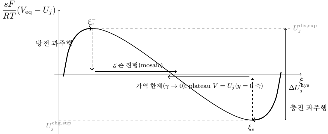
Figure 9: 비단조 평형 전위 (1.67) ( \Omega_j = 4RT )와 과주행 경로 — 극값이 spinodal 에 서는 근거는 식 (1.68). 방전(굵은 경로, 좌상)은 상승 준안정 가치를 타고 극대 \xi_s^- 까지 과주행한 뒤, 분리가 점화되며 공존 plateau ( V = U_j , y = 0 축)로 낙하해(점선 화살표) mosaic 공존으로 진행한다. 충전(우하)은 거울상으로 극소 \xi_s^+ 까지 과주행한다. 두 극값의 차가 spinodal 상한 gap \Delta U_j^{\text{hys}} 이고(위첨자 sup는 spinodal 상한 표시), 실측 분기는 축소 인자 \gamma_j 만큼 그 안쪽에 선다 — \gamma \rightarrow 0 의 가역 한계에서 두 경로가 모두 y = 0 의 plateau 로 합쳐진다.
