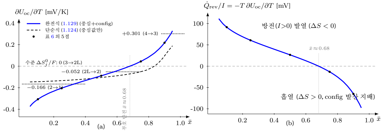
Figure 22: 완전식이 만드는 하프셀 엔트로피 계수와 가역 발열의 실제산 곡선 — 좌표는 식 그대로의 수치 평가다(4-전이 staging 입력: 표 3의 \Delta S_j^0 , w_j = RT/F ( n_j=1 ), 298.15 K; 각 \bar{x} 에서 전하 보존 음함수 (1.119)를 풀어 U_{oc} 를 얻은 뒤 평가). (a) \partial U_{oc}/\partial T(\bar{x}) — 파란 실선 = 완전식 (1.129)(중심 표준값+분포 config), 검은 파선 = 단순식 (1.124)(중심값만) 이고 둘의 차가 봉우리 내부 config 항이다(파생 B). 점선 수평선은 전이별 수준 \Delta S_j^0/F — 곡선이 전이 경계마다 계단 없이 인접 수준 사이를 연속으로 지난다(파생 A의 연속 블렌드). ●는 표 6의 다섯 점과 일치하며 \bar{x} \approx 0.25 값이 계산 예제 (§1.18.2)의 -0.204 / 단순식 -0.134 mV/K 다. (b) 가역 발열 \dot{Q}_{rev}/I = -T\partial U_{oc}/\partial T (식 (1.128)) — \bar{x} \approx 0.68 에서 방전 발열이 흡열로 스스로 반전한다(임의 함수·외부 스위치 없이 분포만으로). 완전식 곡선은 폭의 열적 서식 w_j = n_j RT/F 를 전제하며, 실측 폭이 T -동결에 가까우면 단순식이 보수적 기준이다 (§1.15.4).
