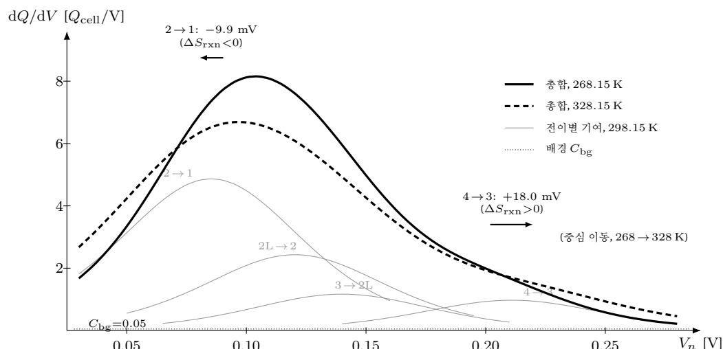
Figure 18: 합산식 (1.101) 이 내는 전체 곡선 — 좌표는 식 그대로의 수치 평가다: 초기 상태의 평형 중 전용 극한( L_V \rightarrow 0, \gamma_j = 0, R_n = 0 )에서 dQ/dV = C_{bg} + \sum_j Q_j \xi_{eq,j}(1 - \xi_{eq,j})/w_j 를 표 2 초기값으로 평가했다( U_j(T) = (-\Delta H_{rxn,j} + T\Delta S_{rxn,j})/F 를 온도마다 재평가, w_j = RT/F - n_j = 1 균일, 배경은 상수 예시 C_{bg} = 0.05 Q_{cell}/V ). 회색 가는 곡선이 298.15 K의 전이별 기여, 굵은 실선. 파선이 268.15/328.15 K의 총합이다. 온도가 오르면 (i) 폭 w = RT/F 가 비례해 열려 봉우리가 낮고 넓어지고(면적 Q_j 보존), (ii) 중심은 \partial U_j/\partial T = \Delta S_{rxn,j}/F 를 따라 전이마다 반대 방향으로 움직인다 — 60 K 동안 2 \rightarrow 1 ( \Delta S_{rxn} = -16 J/(mol K))은 -9.9 mV로 왼쪽, 4 \rightarrow 3 (+29)은 +18.0 mV로 오른쪽(화살표), 3 \rightarrow 2 L(0)은 제자리다. 다운도 피팅에서 온도마다 U_j(T) 를 따로 읽어야 하는 까닭 (§1.3)이 이 한 장이다.
