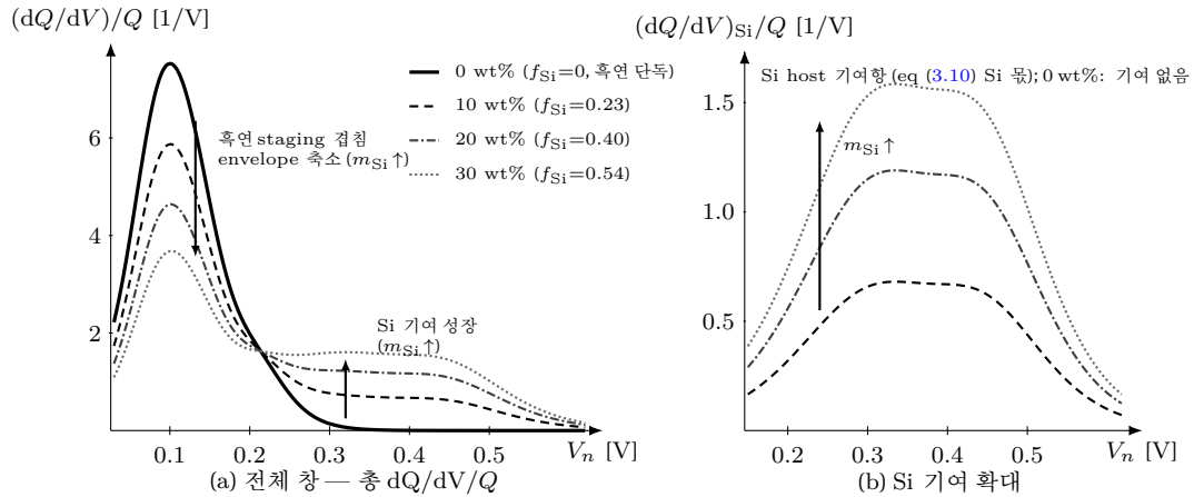
Figure 2: 블렌드 f_{\text{Si}} (wt% 스왑) 가중 평균 dQ/dV — 좌표는 원소 Si (elemental) host 블렌드의 평형 식 (3.10) 실제산이다. 그 |I| \rightarrow 0 중 \sum_{\text{host}} \sum_j Q_j^{\text{host}} \xi_{\text{eq},j}^{\text{host}} (1 - \xi_{\text{eq},j}^{\text{host}}) / w_j^{\text{host}} 을 T=298.15 \text{ K} \cdot C_{\text{bg}}=0 에서 평가하고 총용량 Q=Q_{\text{gr}}+Q_{\text{Si}} 로 정규화했다(곡선 아래 면적 = 1 규약, 곡선당 ~53–66 표본점). 질량↔용량 환산은 §3.3.1 각주의 환산 규약 f_{\text{Si}} = m_{\text{Si}} q_{\text{Si}} / [m_{\text{Si}} q_{\text{Si}} + (1 - m_{\text{Si}}) q_{\text{gr}}] ( q_{\text{Si}}=1000 \text{ mAh/g} 원소 Si 1차 가역[2], tier-A· q_{\text{gr}}=372 )로, m_{\text{Si}}=0/10/20/30 \text{ wt\%} \Rightarrow f_{\text{Si}}=0/0.230/0.402/0.535 ( Q=0.97/1.26/1.62/2.09 Q_{\text{cell}} ). (a) 전체 창: 흑연 staging 4-peak 겹침 envelope 는 m_{\text{Si}} 증가로 정규화 높이가 7.5 \rightarrow 3.7 [1/V] 로 축소하고 ( Q_{\text{gr}} 절대값은 불변이나 총용량 Q 가 커져 상대 몫 1-f_{\text{Si}} 로 줄어듦), 원소 Si 두 경사 전이(중심 0.30/0.45 V, 폭 0.060/0.050 V)의 기여가 고전위 쪽에서 성장해 V_n \approx 0.26 \text{ V} 부근에서 순서가 역전한다. (b) 그 Si host 몫만 떼어 확대: 0 \rightarrow 1.585 [1/V] 로 자란다( f_{\text{Si}} 에 정비례). 곡선 개형(전이 중심·폭)은 원소 Si 평균 전위대 0.2–0.5 V[10](tier-B) 안의 tier-C 시연값이며(신뢰값 아님, 피팅 override 전제), 원소 Si (elemental) 케이스는 \text{SiO}_x 절대전위 같은 “확인 필요” 공백을 쓰지 않는다. f_{\text{Si}} \rightarrow 0 에서 (a)의 실선은 흑연 단독 평형곡선과 부동소수점까지 일치한다(bit-exact, 식 (3.9)); §1.10 그림 18 와 동일 흑연 골격).
