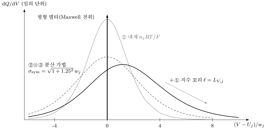
Figure 12: 두-상 broadening 의 폭 예산(식 (1.59); 좌표는 식 그대로의 수치 평가). 평형 델타(수직 화살)에 ② 내재 logistic 미분 중(폭 w_j , 가는 실선)이 없히고, ③ 양상불 \eta 산포와의 합성곱이 분산 가법으로 종을 넓히며(예시 \sigma_\eta = 1.25w_j — 유효 scale \sqrt{1 + 1.25^2} w_j \approx 1.6w_j 의 같은 함수축으로 표시, 파선), ① 유한율속이 한쪽 지수 꼬리(예시 L_V = 1.5w_j 와의 단측 합성곱 — 수치 적분)를 늘여 종을 소인 방향으로 민다(굵은 실선). 대칭 두 뚫은 w_j 하나에 흡수되고 비대칭 꼬리만 L_{V,j} 로 분리된다.
