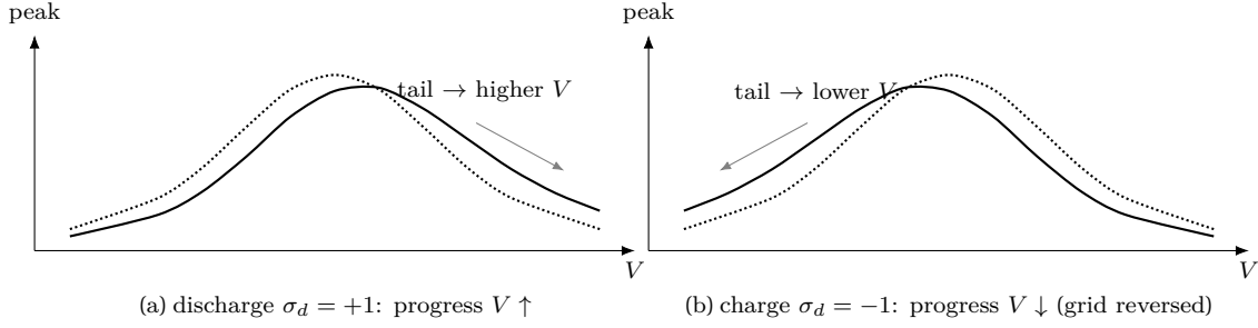
Figure 15: 인과 꼬리의 방향. 점선 = 평형 종( \xi_{eq}(1 - \xi_{eq})/w , 방향 불변). 실선 = peak_shape with tail. (a) 방전은 진행이 V \uparrow 라 꼬리가 높은 V 쪽으로 늘어진다(격자 그대로). (b) 충전은 진행이 V \downarrow 라 격자를 뒤집어 필터한 뒤 되돌려(역순 저역통과의 재역순) 꼬리가 낮은 V 쪽으로 — 방전의 거울. 두 경우 모두 peak 는 양수.
