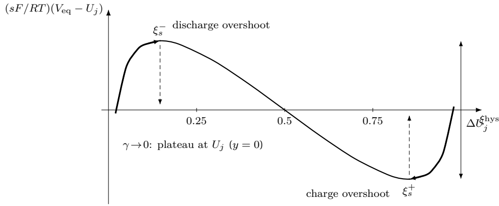
Figure 8: 비단조 평형 전위 V_{eq}(\xi) (식 (1.44), \Omega_j = 4RT — 좌표는 식 그대로의 수치 평가)와 과주행. 방전(굵은 경로, 좌상)은 극대 \xi_s^- 까지, 충전(우하)은 극소 \xi_s^+ 까지 과주행해 중심이 갈라진다. 두 극값 차가 spinodal 상한 gap \Delta U_j^{\text{hys}} (식 (1.47)), 실측 분기는 \gamma_j 만큼 안쪽(식 (1.49)). \gamma \rightarrow 0 가역 한계에서 두 경로가 y = 0 plateau 로 합쳐진다.
