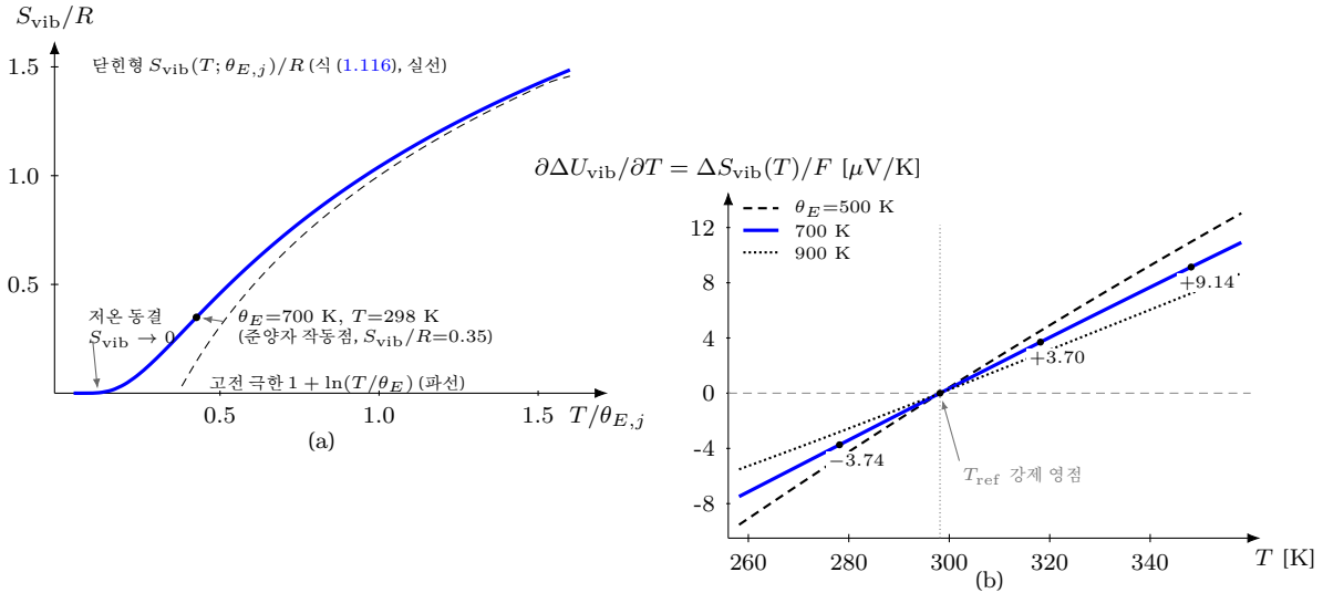
Figure 20: Einstein 진동 보정의 두 얼굴 — 좌표는 식 (1.116)·(1.118) 그대로의 수치 평가다. (a) 단원형 S_{\text{vib}}(T; \theta_{E,j})/R : 저온( u_j \rightarrow \infty )에서 0 으로 동결되고 고전 극한(파선) 1 + \ln(T/\theta_E) 에 T/\theta_E \gtrsim 1 에서 붙는다 — 앞 절이 중심 표준값에 흡수한 “ T -무관 상수”는 이 곡선을 T_{\text{ref}} 에서 한 번 평가해 동결한 값이다. ● 는 \theta_E = 700 \text{ K} · 298 \text{ K} 의 준양자 작동점. (b) 중심 이동의 온도 기울기 \partial \Delta U_{\text{vib}} / \partial T = \Delta S_{\text{vib}}(T)/F : \theta_E = 500/700/900 \text{ K} 모두 T_{\text{ref}} 의 강제 영점을 지나 로그형 곡률로 자라며, ● 는 본문 §1.14.3 의 수치 ( \theta_E = 700 \text{ K} 에서 -3.74/0/+3.70/+9.14 \mu\text{V/K} )다. electronic 항( \propto T )은 곡률이 0 이라 두 함수형이 다운도 곡률 피팅에서 갈리고, 분리에는 준양자 영역에 놓인 온도점 셋 이상이 필요하다.
