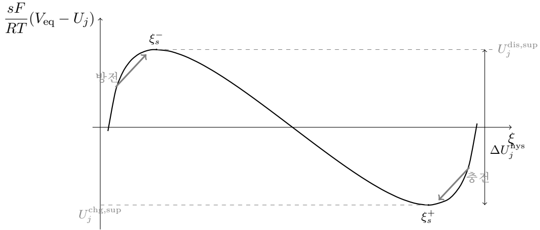
Figure 8: 비단조 평형 전위 (1.63) ( \Omega_j = 4RT ). 방전은 상승 준안정 가지를 타고 극대 \xi_s^- 까지, 충전은 반대쪽 극소 \xi_s^+ 까지 과주행한다. 두 극값의 차가 spinodal 상한 gap \Delta U_j^{\text{hys}} 이고 (위 첨자 sup 는 spinodal 상한 표시), 실측 분기는 축소 인자 \gamma_j 만큼 그 안쪽에 선다.
