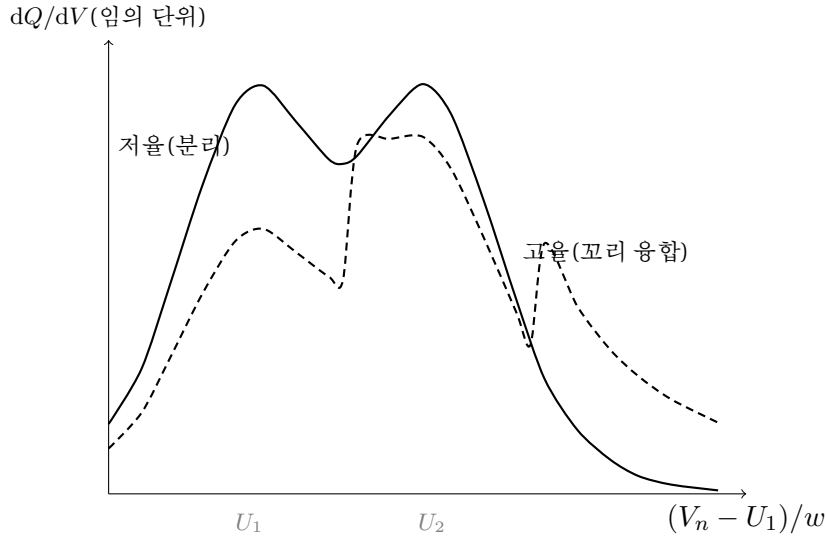
Figure 7: 두 인접 전이의 융합(중심 간격 3.9w ). 실선은 저율( r_a \rightarrow 0 ) — 골이 깊어 분리가 일어난다. 파선은 고율( r_a = 0.35 , L_V = 4w ) — 식 (1.62) 그대로, 중 향이 (1 - r_a) = 0.65 로 깎이고 각 전이의 꼬리가 다음 전이 쪽으로 뻗어 골의 우측을 메우고 뒤 어깨를 들어 올리므로 분리 판독이 지워진다. 저온도 같은 방향으로 작용한다.
