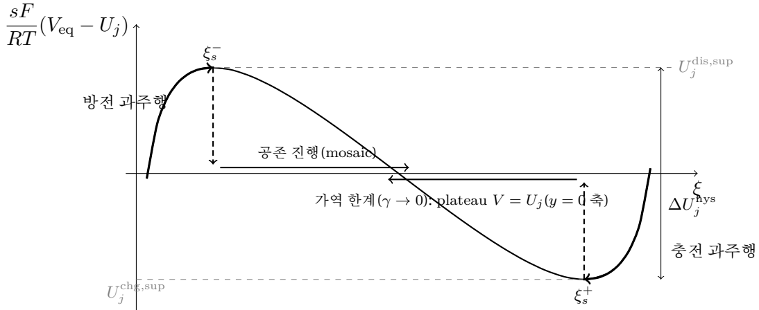
Figure 9: 비단조 평형 전위 (1.71) ( \Omega_j = 4RT )와 과주행 경로 — 극값이 spinodal 에 서는 근거는 식 (1.72). 방전(굵은 경로, 좌상)은 상승 준안정 가치를 타고 극대 \xi_s^- 까지 과주행한 뒤, 분리가 점화되며 공존 plateau ( V = U_j, y = 0 축)로 낙하해(점선 화살표) mosaic 공존으로 진행한다. 충전(우하)은 거울상으로 극소 \xi_s^+ 까지 과주행한다. 두 극값의 차가 spinodal 상한 gap \Delta U_j^{\text{hys}} 이고(위첨자 sup 은 spinodal 상한 표시), 실측 분기는 축소 인자 \gamma_j 만큼 그 안쪽에 선다 — \gamma \rightarrow 0 의 가역 한계에서 두 경로가 모두 y = 0 의 plateau 로 합쳐진다.
