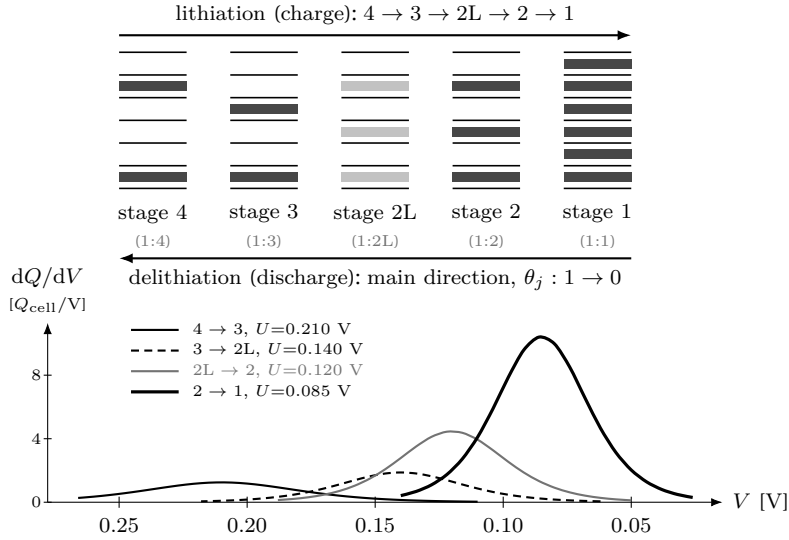
Figure 2: 흑연 staging 의 갤러리 채움 도식(위)과 대응 dQ/dV peak(아래, 식 (1.56) 의 초기값 수치 평가 — dQ/dV = Q_j \xi_{eq}(1 - \xi_{eq})/w_j , 표 2 의 U_j, Q_j, w_j ). 위: 수평선이 그려진 층, 음영 띠가 리튬이 든 층간 갤러리다. 채울수록 stage 번호가 줄어 stage 1(LiC 6 , 완전 채움)에 닿고, 열 아래 비율(1:4→1:1) 이 각 stage 의 갤러리 점유 주기다. stage 2L 은 면내 질서가 풀린 단계라 열게 표시했다. 아래: 네 초기값 전이의 실제 peak — 높이 Q_j/(4w_j) 는 전이마다 크게 다르다 (2 → 1 이 가장 큼, 10.4 Q_{cell}/V ). 주의 — 위 갤러리 열 간격은 범주형(등간격 스케치)이고 아래 V 축은 실제 전위 스케일(비등간격 — 3 → 2L 과 2L → 2 은 겨우 20 mV 차이로 갤러리 열 간격에 선형 정렬되지 않는다)이라, 둘은 전이명 (예 2 → 1)으로만 대응시킨다. 본 문건 방향은 방전(탈리튬화)이다.
