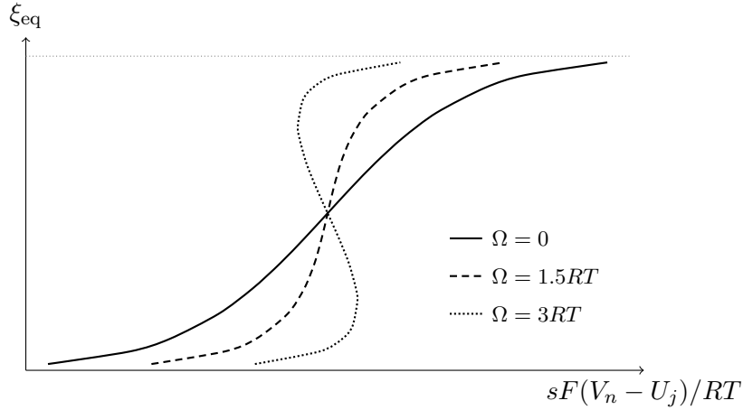
Figure 2: 평형 등온선 (1.19) 의 한 모수축. \Omega = 0 (실선)은 폭 RT/F 의 logistic, \Omega = 1.5RT (파선)는 중심이 가팔라진(좁아진) 단조 곡선, \Omega = 3RT > 2RT (점선)는 비단조 — 한 전위에 세 \xi 가 대응한다. 단조에서 비단조로 넘어가는 경계가 \Omega = 2RT , 곧 임계 온도 T_{c,j} = \Omega_j/2R 다.
