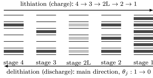
Figure 2: 흑연 staging의 갤러리 채움 도식. 수평선이 그래핀 층, 음영 띠가 리튬이 든 층간 갤러리다. 채울수록 stage 번호가 줄어 stage 1(LiC 6 , 완전 채움)에 닿고, 각 stage 전이가 dQ/dV 에 peak 하나를 남긴다. stage 2L은 면내 질서가 풀린 단계라 열게 표시했다. 코드의 전이 리스트 4건이 이 전이들의 초기값이며( U \approx 0.21/0.14/0.12/0.085 V), 본 문건 방향은 방전(탈리튬화)이다.
