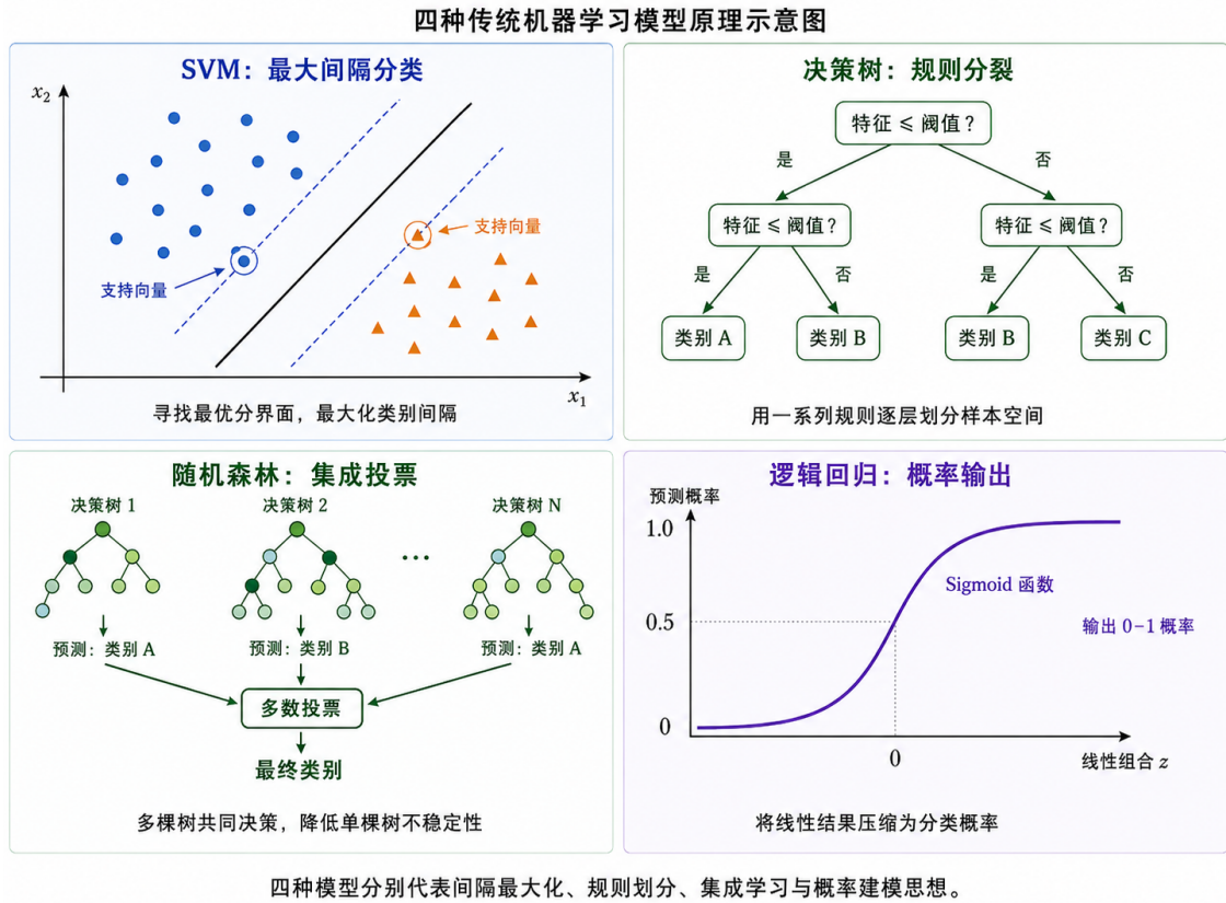
图 2.1 四种传统机器学习模型原理示意：间隔最大化、规则分裂、集成投票与概率输出
