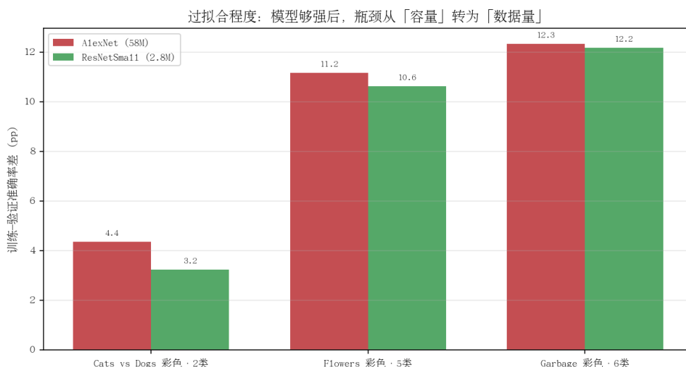
图 6.7 AlexNet 与小型 ResNet 的过拟合程度对比（训练-验证准确率差）
