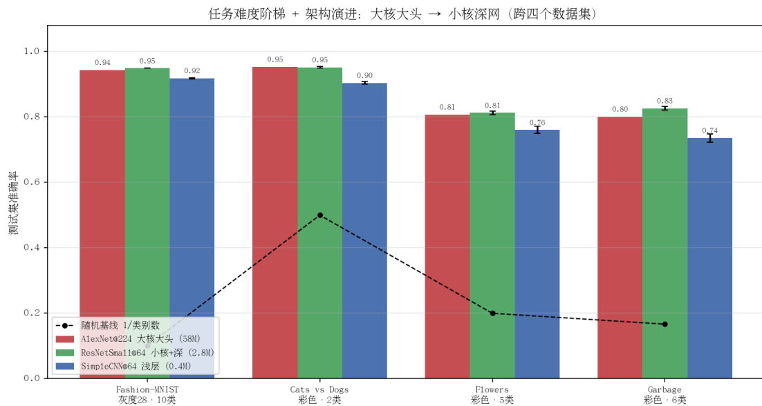
图 6.2 任务难度阶梯与三模型准确率对比（误差棒为多种子标准差）
