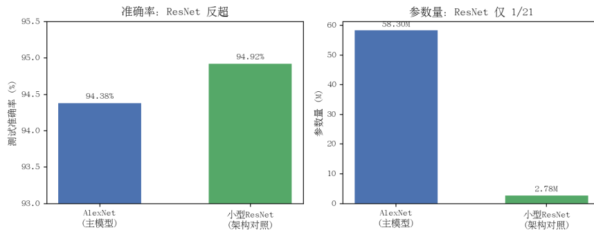
图 5.2 AlexNet 与小型 ResNet 架构对照
