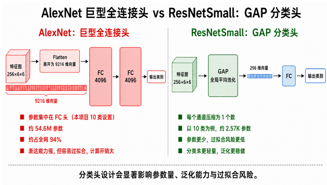
图 6.6 巨型全连接头与全局平均池化头的对比：后者参数少四个数量级、过拟合更轻
