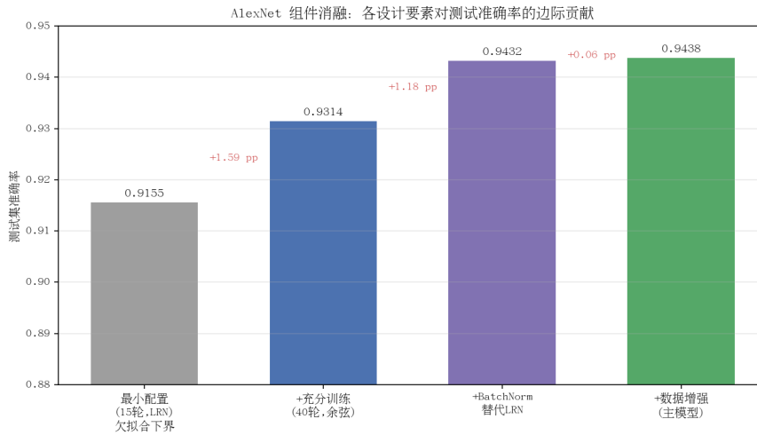
图 5.1 组件消融实验结果对比
