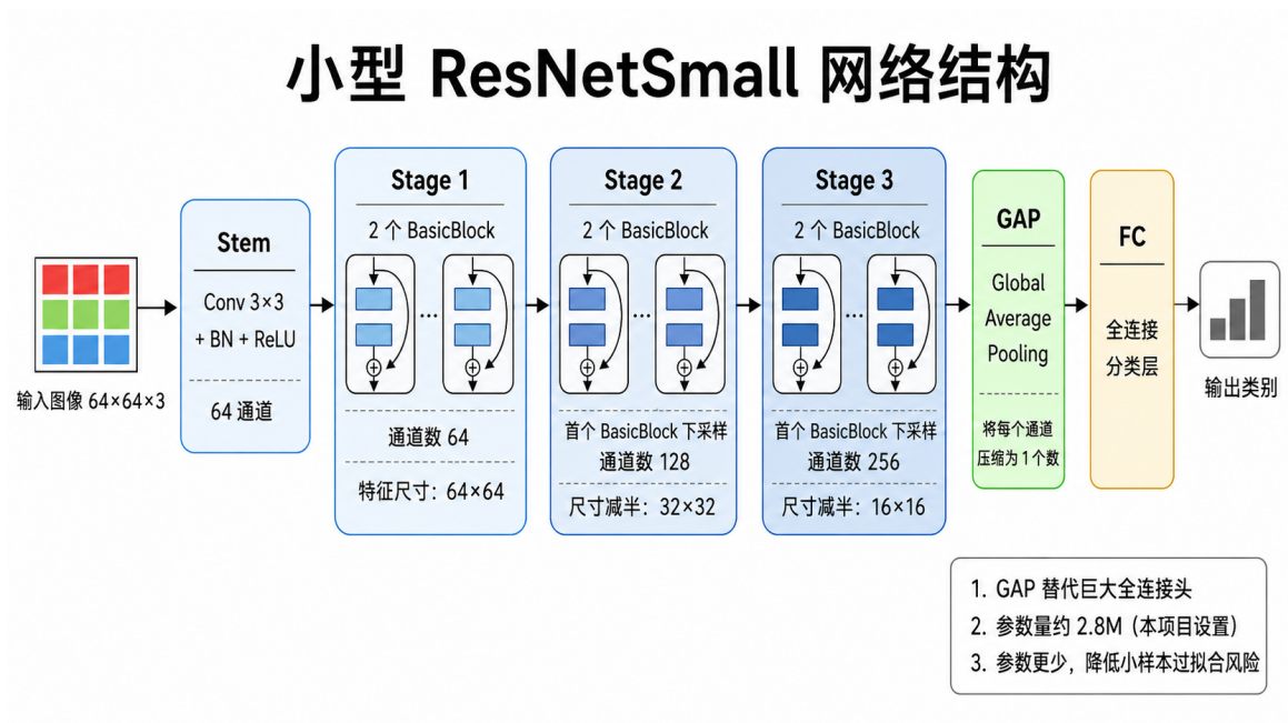
图 6.5 小型 ResNet 整体结构: Stem + 三个 Stage (各含 2 个残差块) + 全局平均池化
