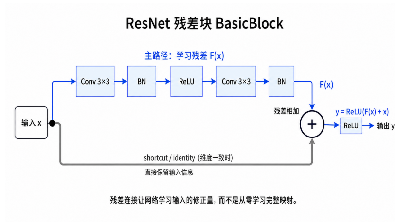
图 6.4 残差块 (BasicBlock) 结构: 捷径使输出为 F(x) + x , 缓解深层退化
