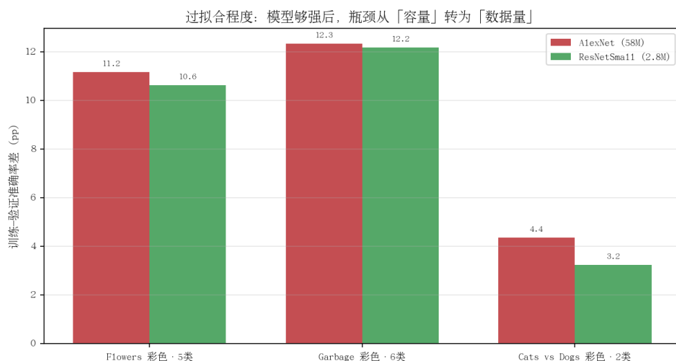
图 6.2 AlexNet 与小型 ResNet 的过拟合程度对比（训练-验证准确率差）
