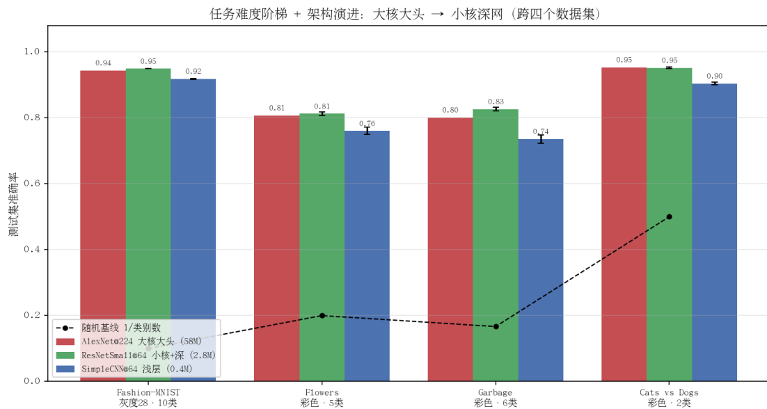
图 6.1 任务难度阶梯与三模型准确率对比（误差棒为多种子标准差）
