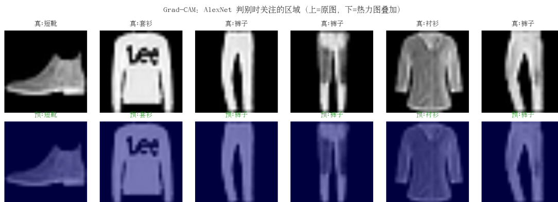
图 5.2 Grad-CAM 可视化: AlexNet 分类时关注的图像区域 (上 = 原图, 下 = 热力图叠加)
