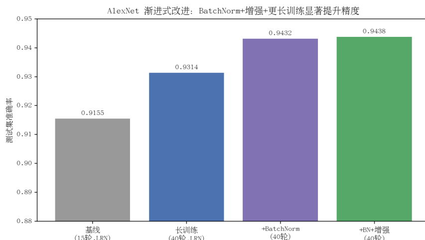
图 5.2 AlexNet 渐进式改进: BatchNorm、数据增强与更长训练显著提升精度
