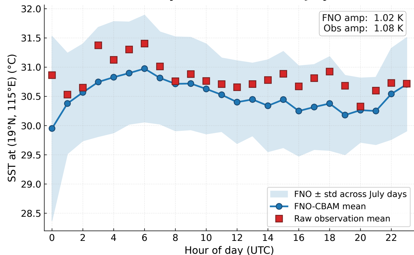
(d) Diurnal cycle at 19°N, 115°E (July 2024)
