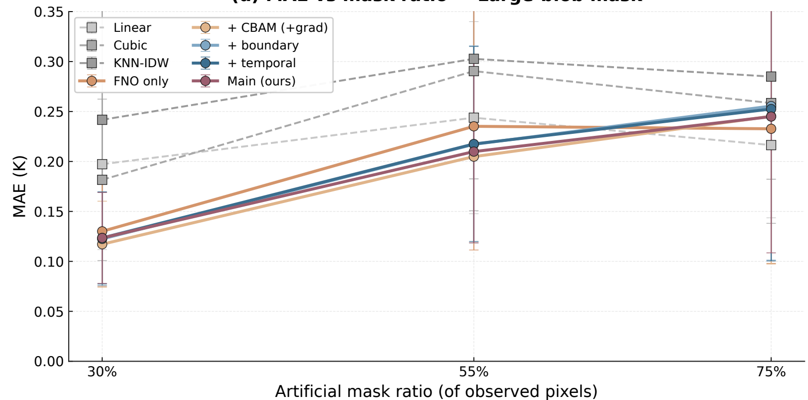
(d) MAE vs mask ratio — Large-blob mask
