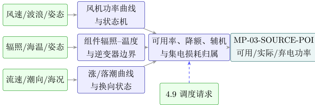
图 4.2 多源能源供给子模型结构
