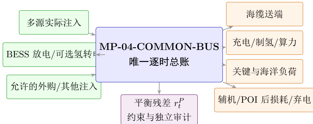
图 4.7 公共母线唯一功率总账结构
