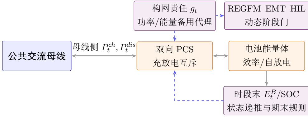
图 4.4 构网型电池储能子模型结构
