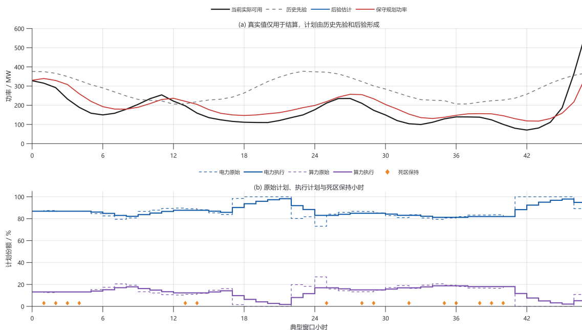
图 5.4 正常典型 48 h 先验-后验功率修正与计划份额防抖
