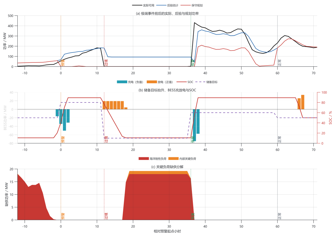
图 5.7 假设台风事件下的后验修正、储备响应与关键负荷缺供
