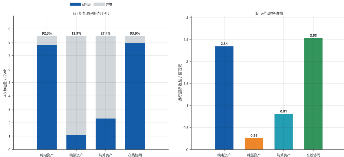
图 5.2 正常典型 48 h 四方案新能源利用及运行层净收益比较
