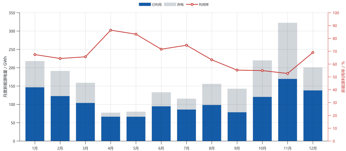
图 5.5 年度逐月新能源利用、弃电与利用率
