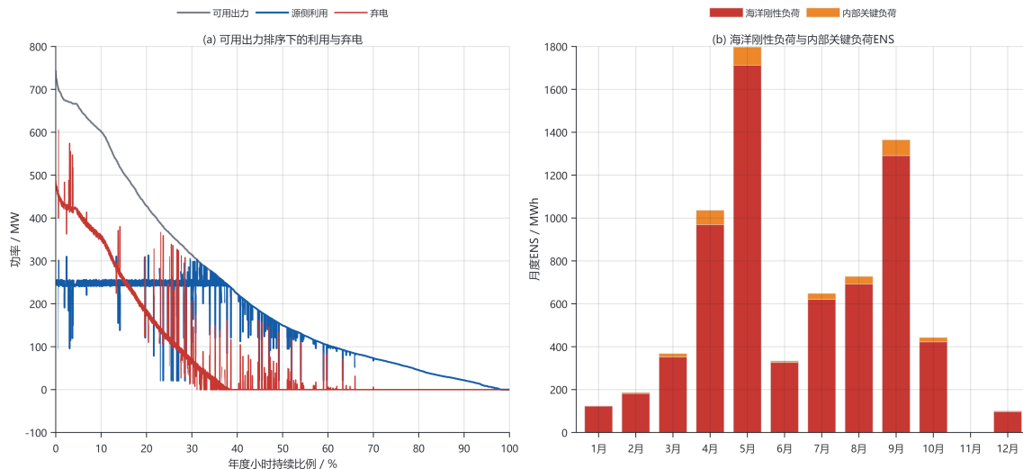
图 5.6 年度出力持续曲线与月度 ENS 构成
