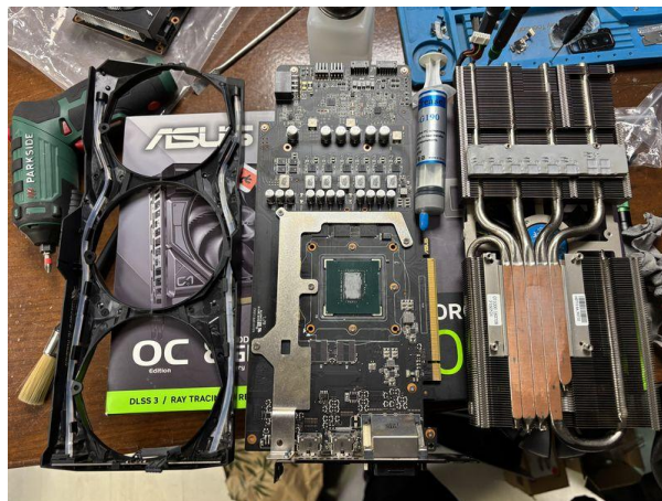
Carte graphique Asus démontée – GPU, radiateur et carrossage séparés
