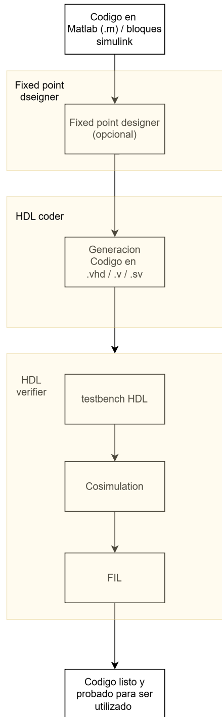
Figura 2.1: Relación entre herramientas de MATLAB para modelado, generación de HDL y verificación en hardware.
