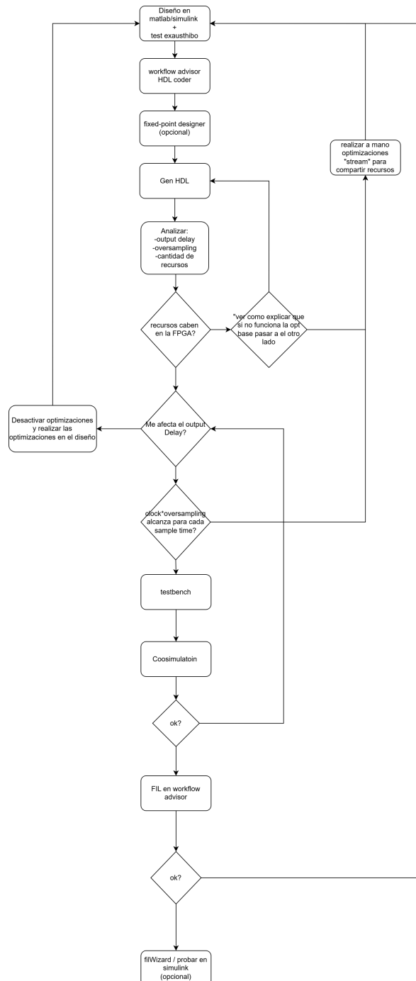
Figura 3.1: Flujo de buenas prácticas para usar HDL Coder en la generación y validación de HDL.
