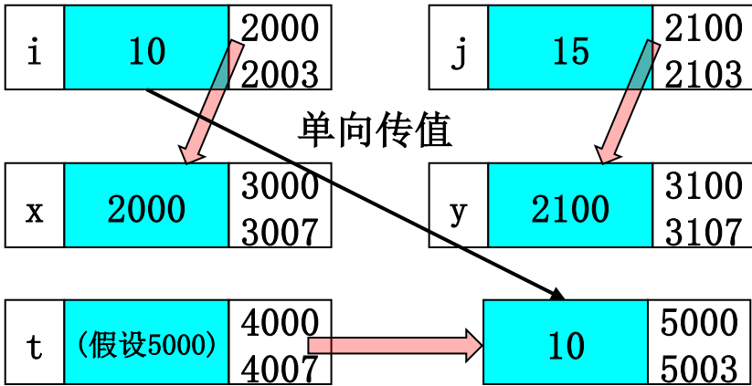
图二 *t = *x;
