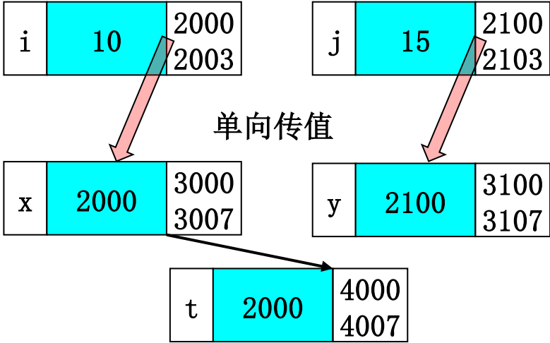
图二 t = x;
