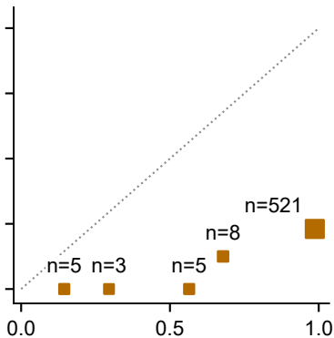
MuSiQue (n=542)
