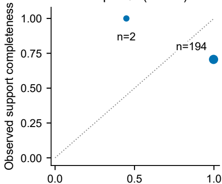
HotpotQA (n=196)
