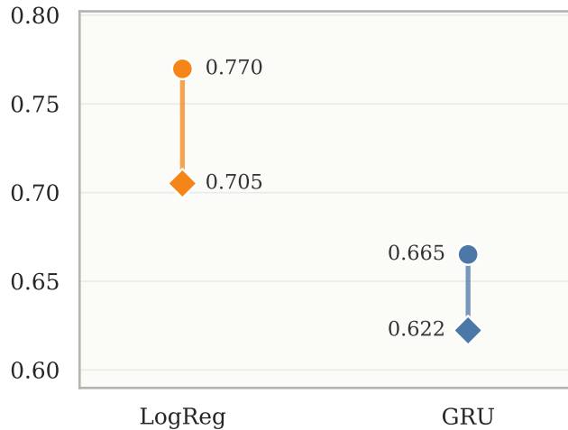
Macro-F1
