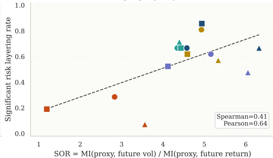
LogReg + post-proc.
