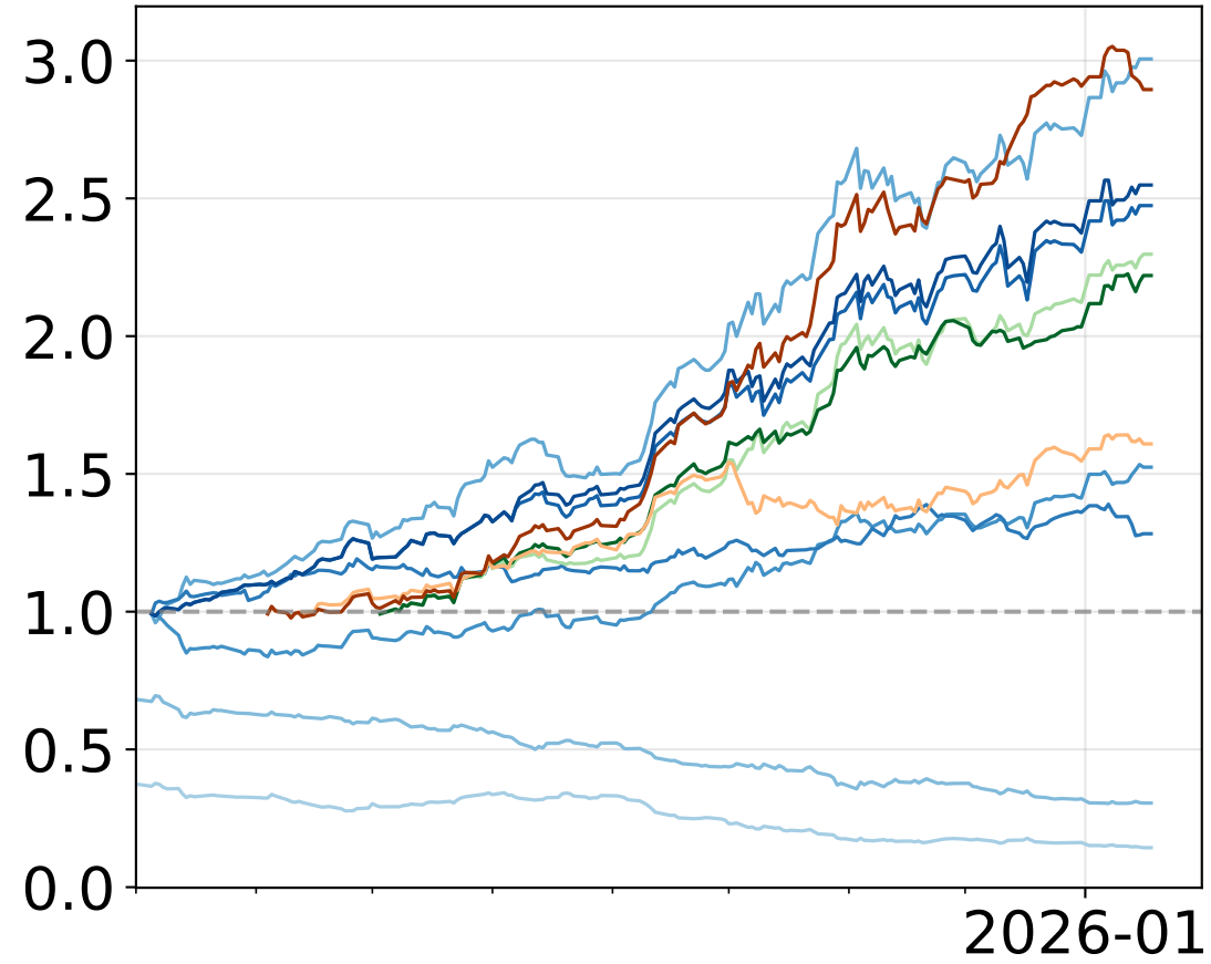
Sortino Mode
