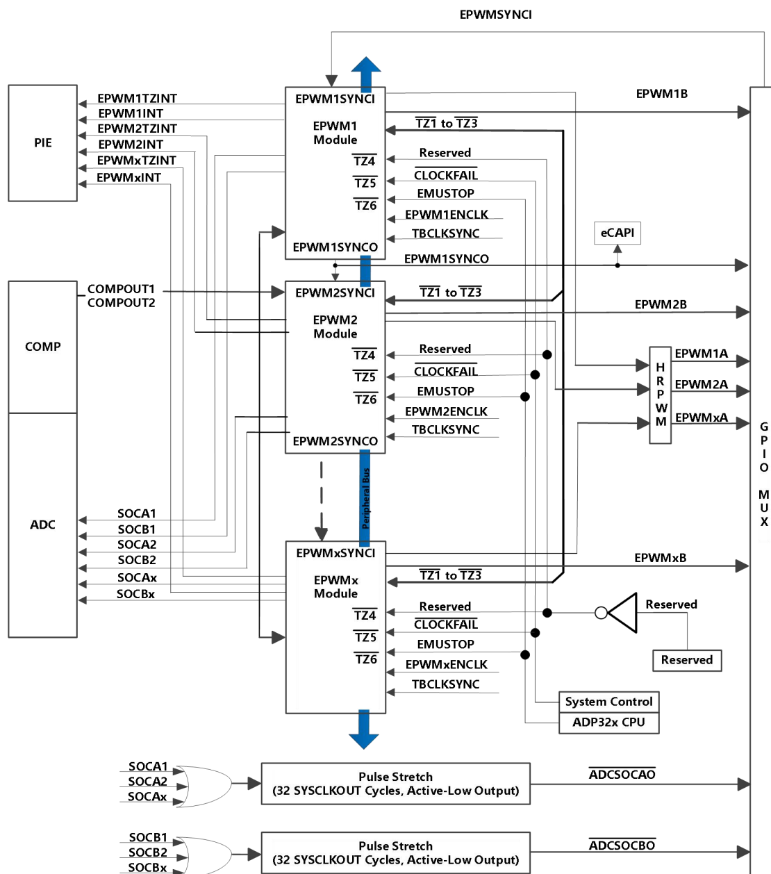
图 4-86 ePWM 框图
