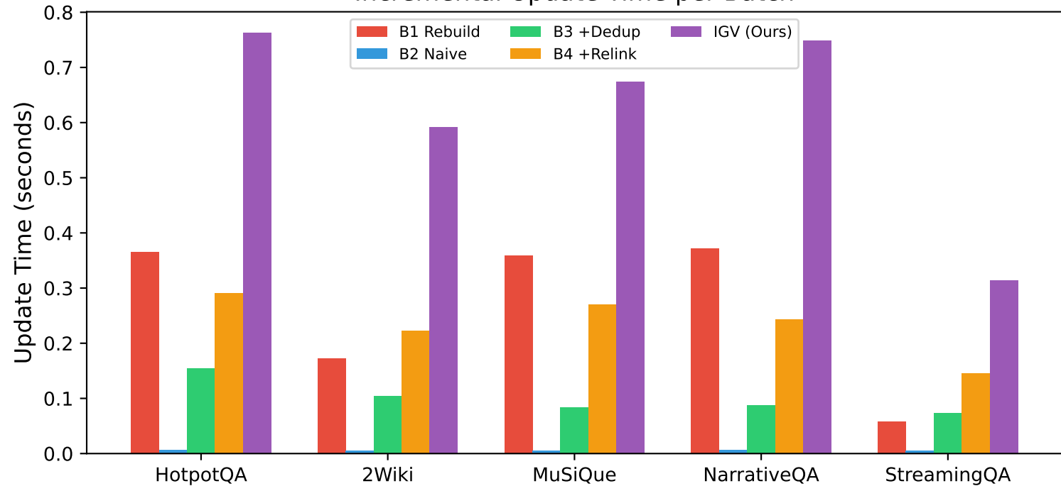
Incremental Update Time per Batch
