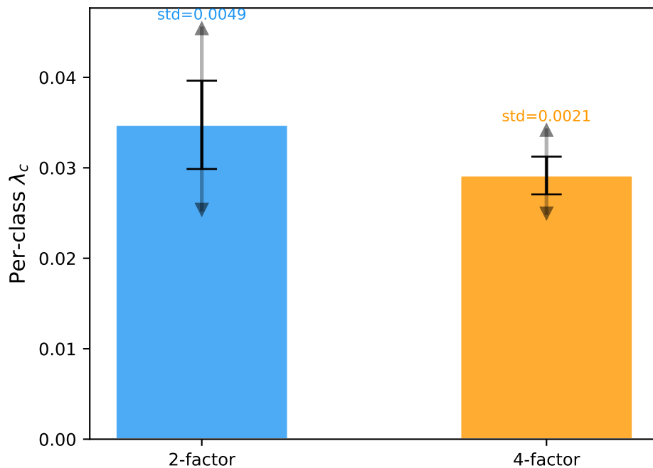
(d) \lambda Distribution (std ratio=2.3 \times )
