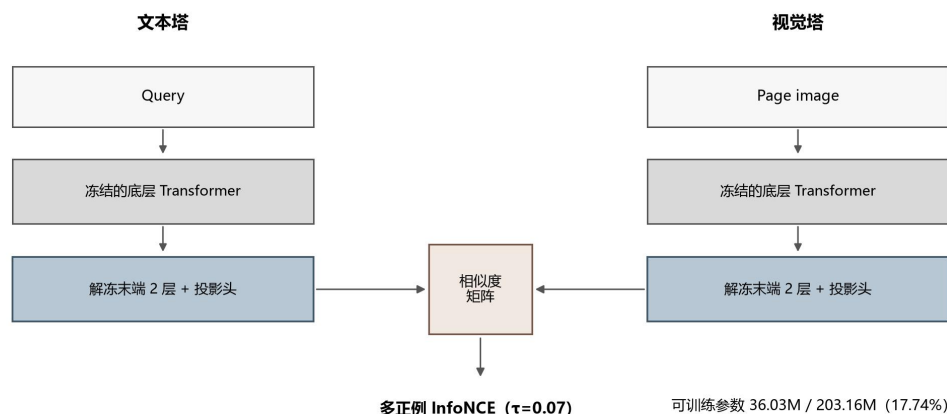
图 4-1 SigLIP 双塔部分微调结构与 InfoNCE 训练目标
