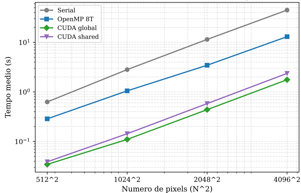
Escalabilidade - Tempo vs tamanho da imagem
