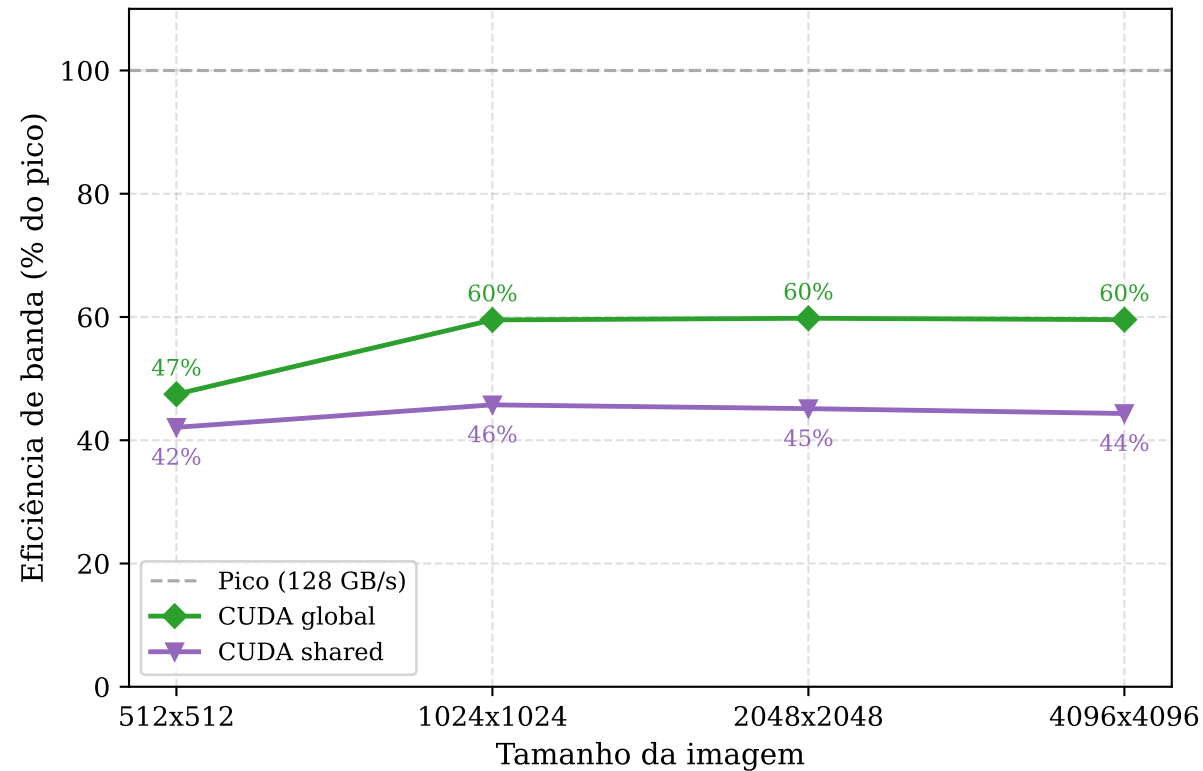
Eficiência de banda de memória da GPU (estimativa, piso)
