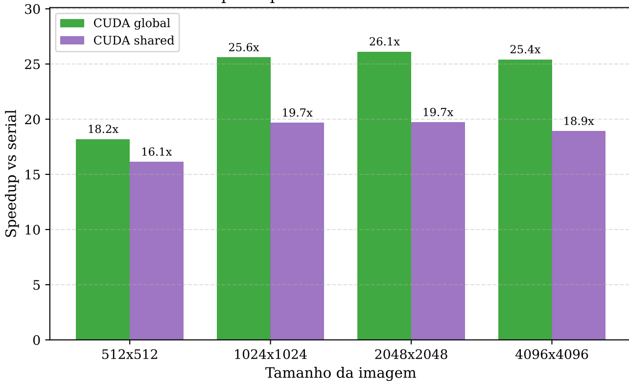
Speedup do CUDA sobre o serial
