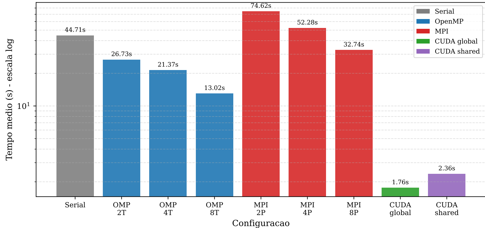
Tempo de execucao - 4096x4096
