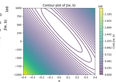
等高线图
