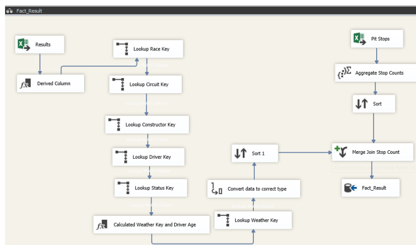
Rysunek 2: ETL dla Fact_Result.
