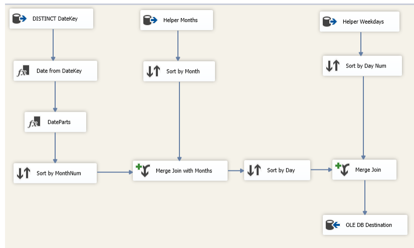
Rysunek 3: ETL dla Dim_Time.
