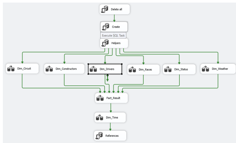
Rysunek 1: Cały ETL.
