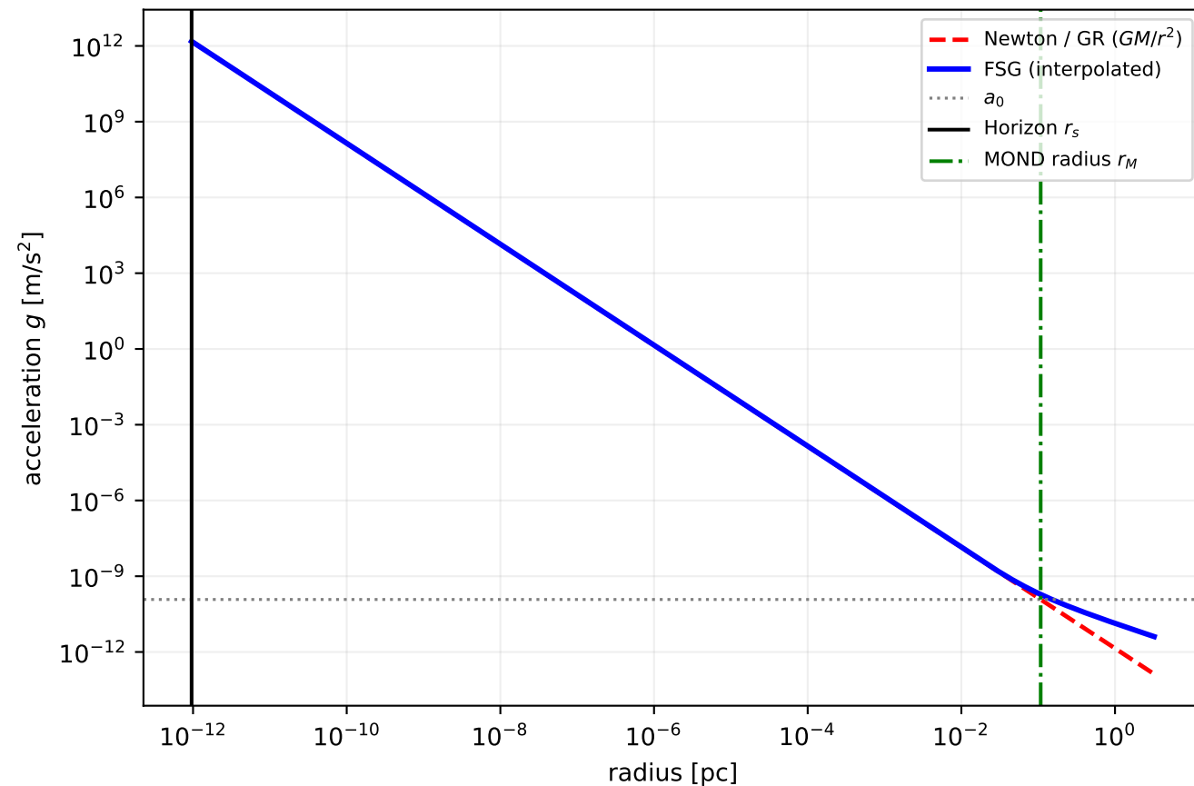
Trou noir stellaire (10 M sun ) r_M/r_s \approx 1e + 11
