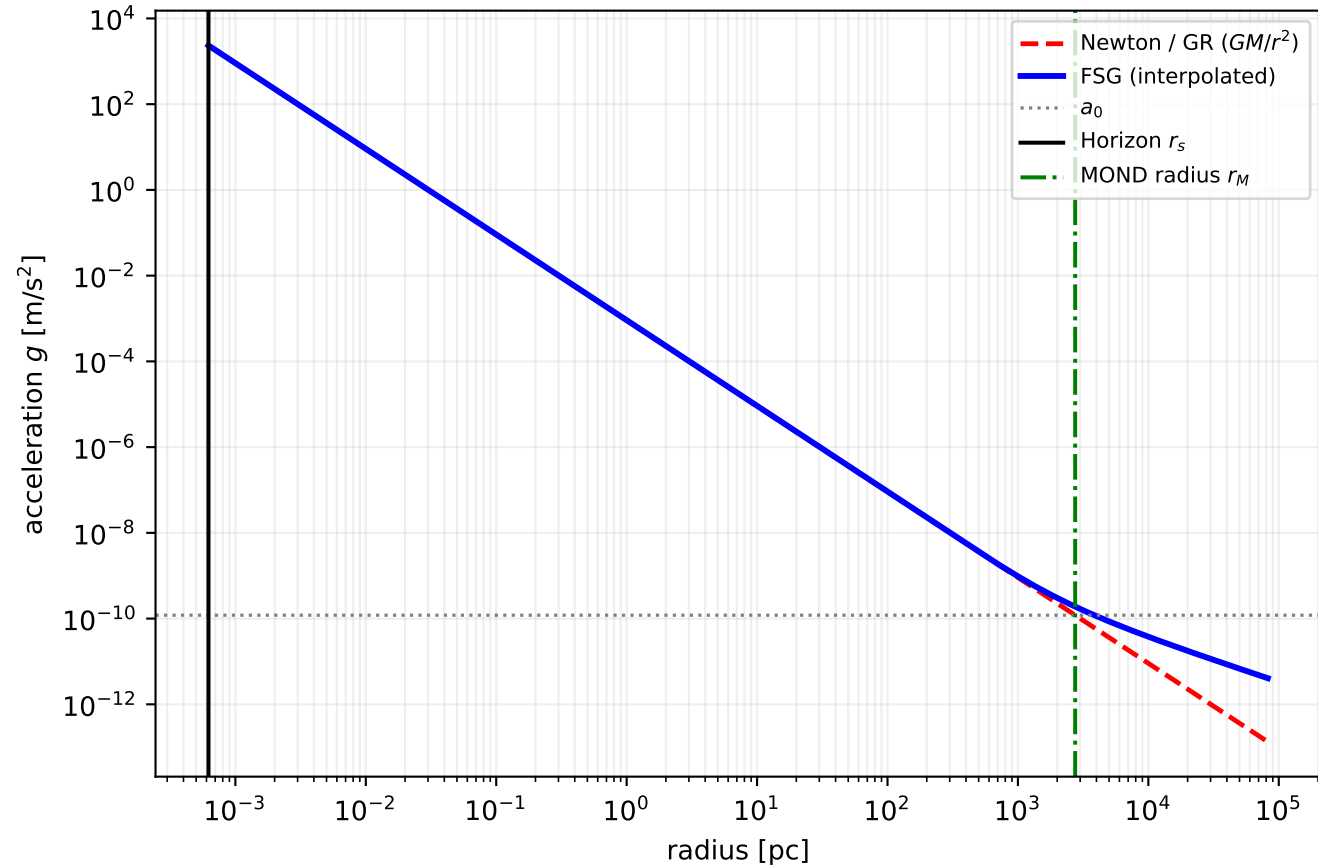
SMBH type M87* (6.5e9 M sun ) r_M/r_s \approx 4e + 06
