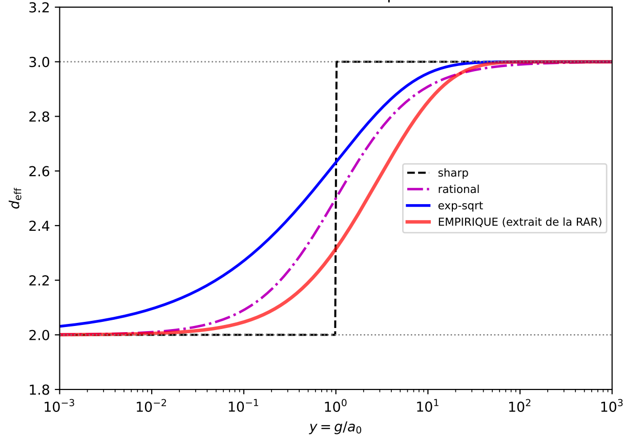
Dimension effective du flux : pilier vs donnees
