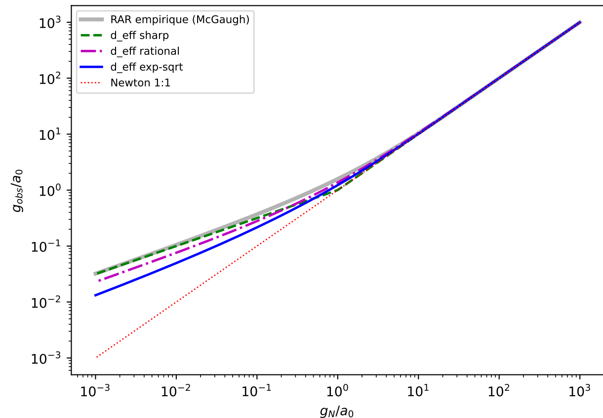
RAR derivée de la loi de flux
