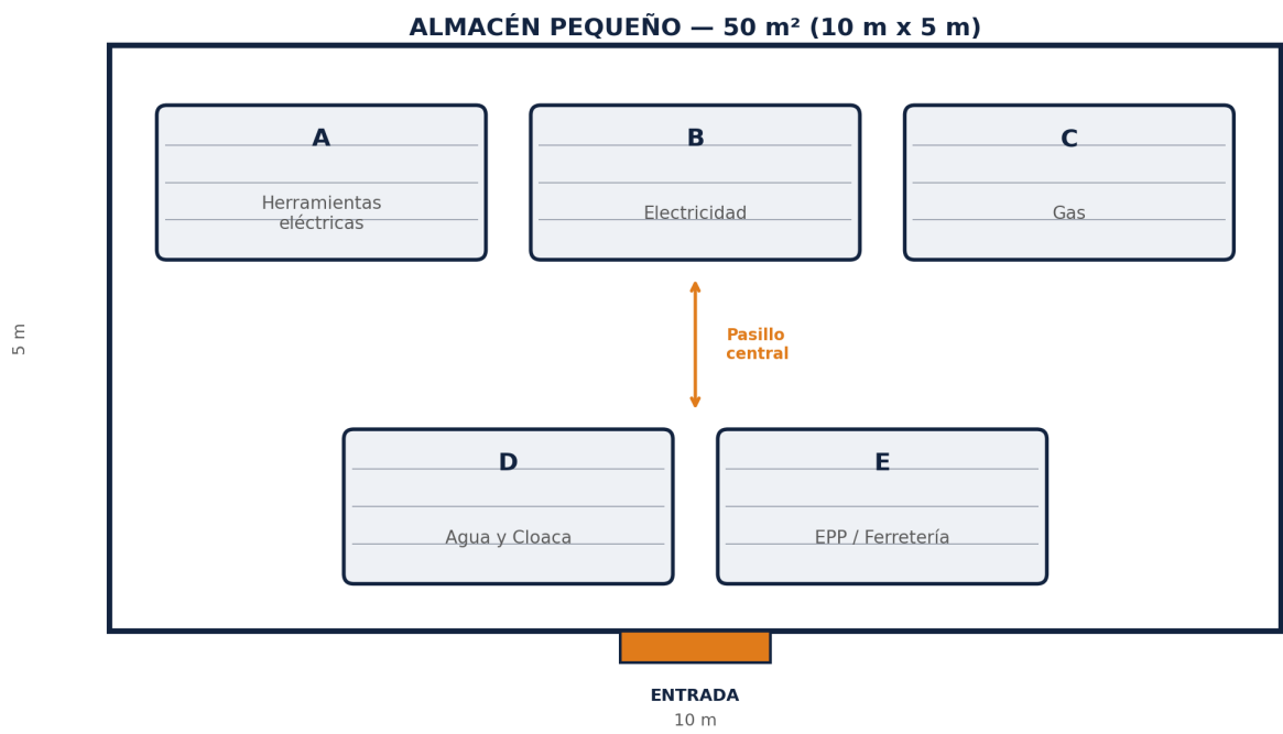
Plano orientativo del almacén con la ubicación propuesta de las 5 estanterías, pasillo central de circulación y entrada.
