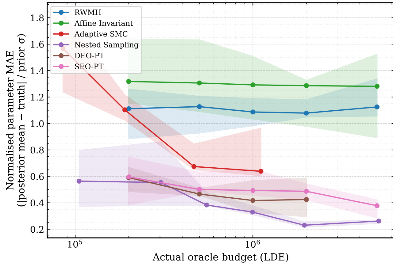
Parameter recovery vs. actual oracle budget
