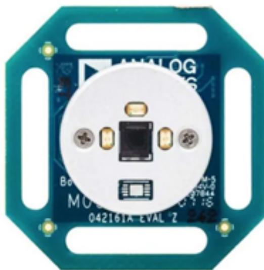
Figura 1.2: Sensor óptico PPG modelo ADPD1081
