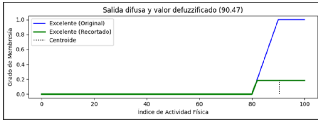
Figura 4.3: Salida difusa del sistema de inferencia donde obtenemos el valor crisp del índice de actividad física resultado del proceso de defuzzificación
