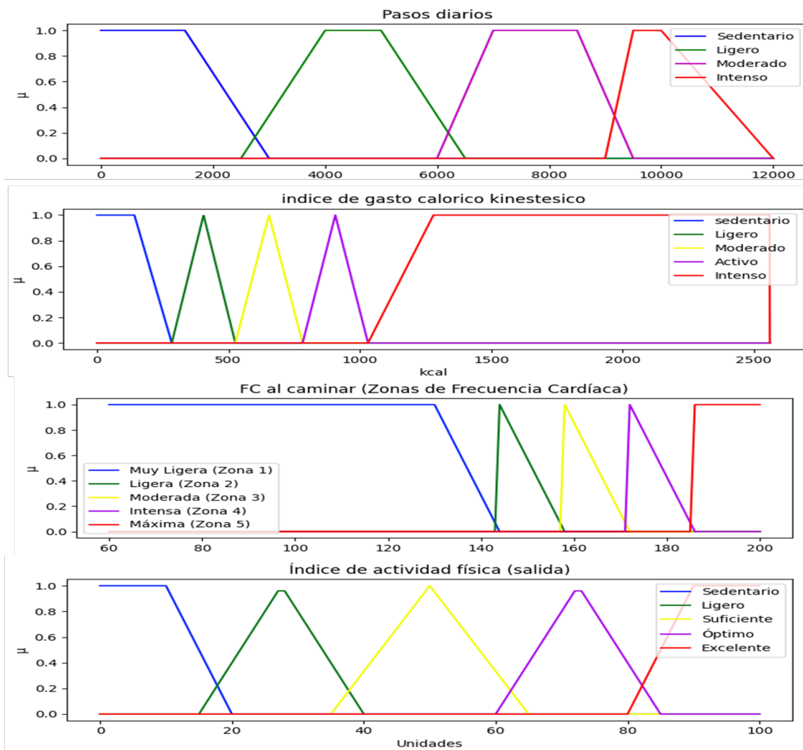
Figura 4.2: Funciones de membresías trapezoidales que representan los universos de discurso: Pasos Diarios, Índice de gasto calórico kinestésico, FC al caminar e índice de actividad física
