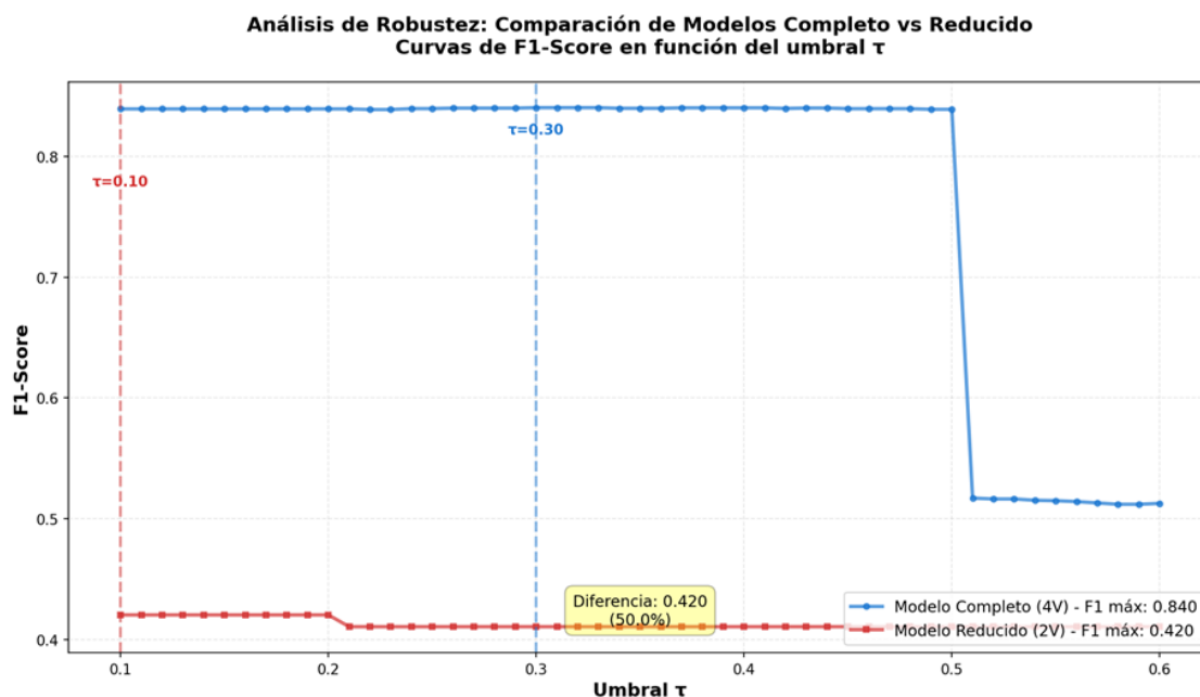
Figura 6.7: Análisis de robustez: Comparación de rendimiento entre Modelo completo (4 variables) y Modelo reducido (2 variables)
