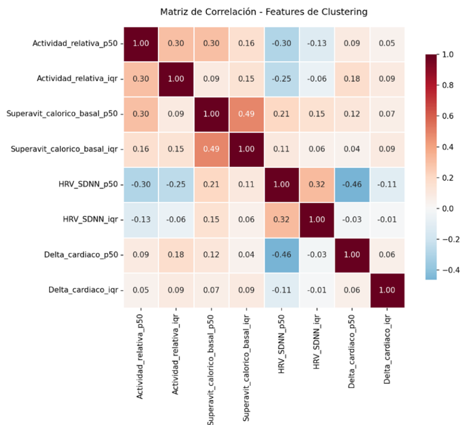
Figura 6.3: Matriz de correlación de características para clustering (verificación de multicolinealidad)
