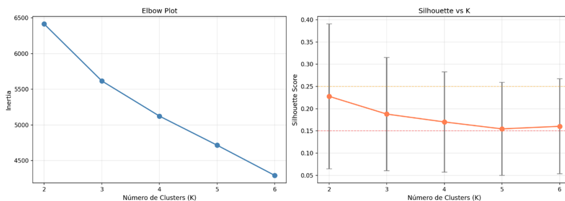
Figura 6.4: Análisis de determinación de K óptimo: Método del codo (Elbow) y Coeficiente de Silhouette
