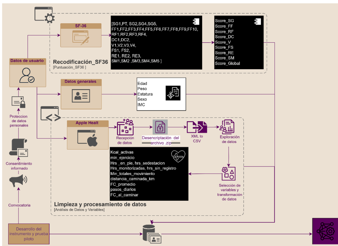
Figura 5.1: Diagrama de flujo del proceso de implementación del proyecto de investigación, desde la obtención de datos hasta la selección, extracción, limpieza y procesamiento de las variables
