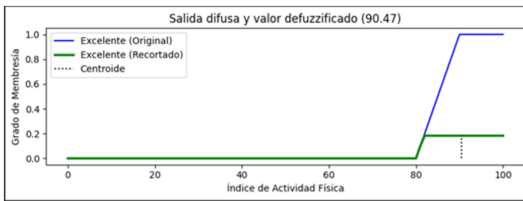
Figura 5.3: Salida difusa del sistema de inferencia donde obtenemos el valor crisp del índice de actividad física resultado del proceso de defuzzificación
