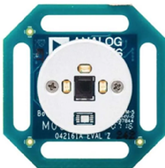
Figura 2.2: Sensor  ptico PPG modelo ADPD1081
