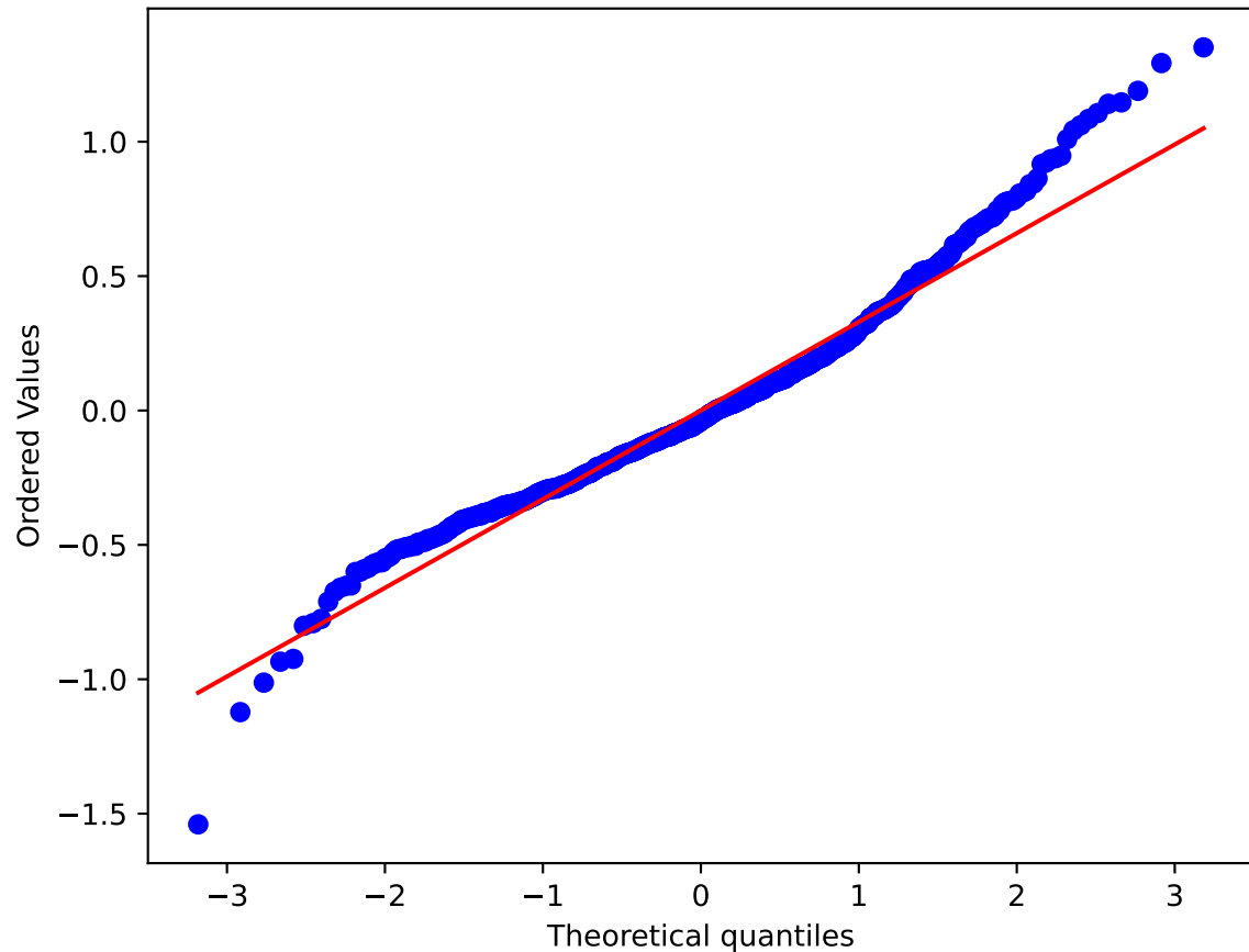
QQ-plot vs Normal (MSAs)
