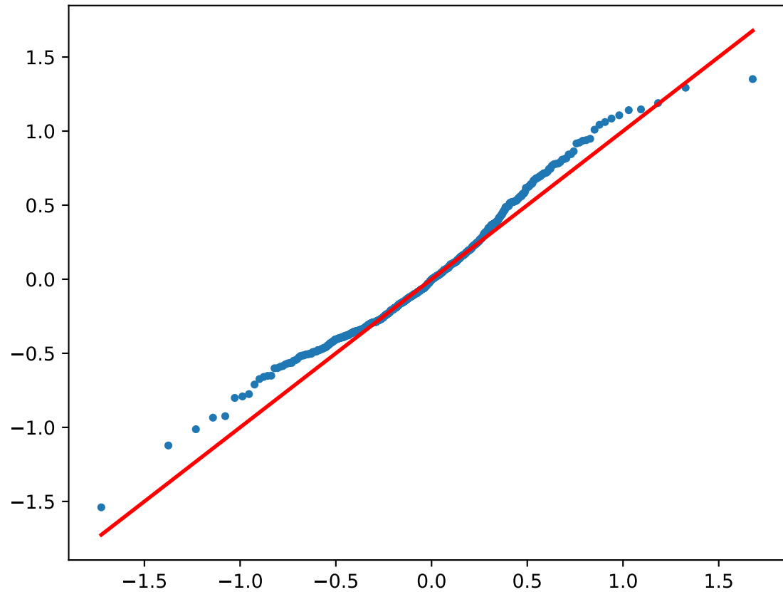
QQ-plot vs Student-t (MSAs)
