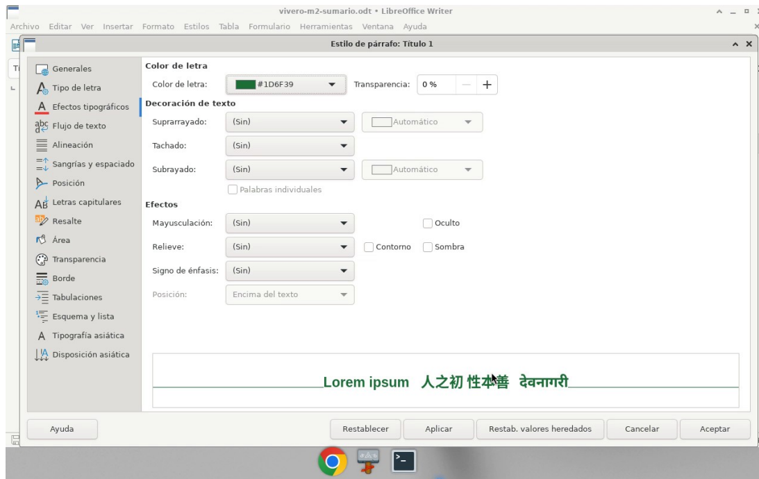
Figura 4. Editar Título 1
