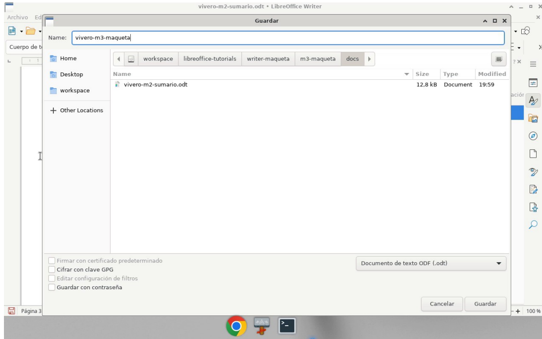
Figura 9. Cierre
