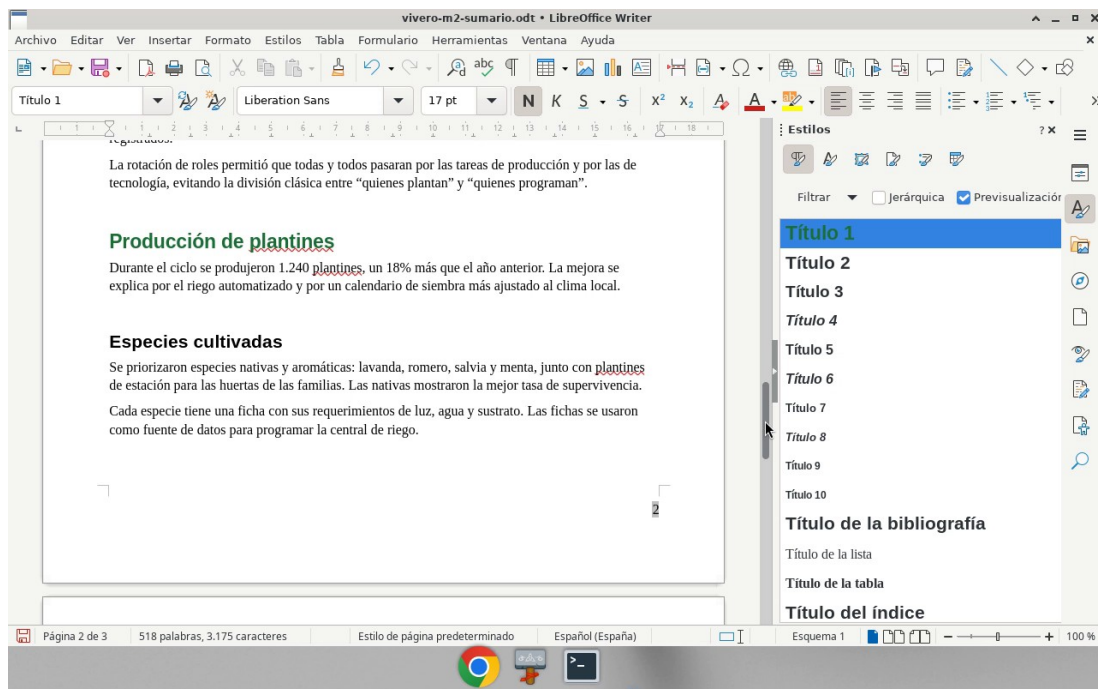
Figura 3. Abrir estilos
