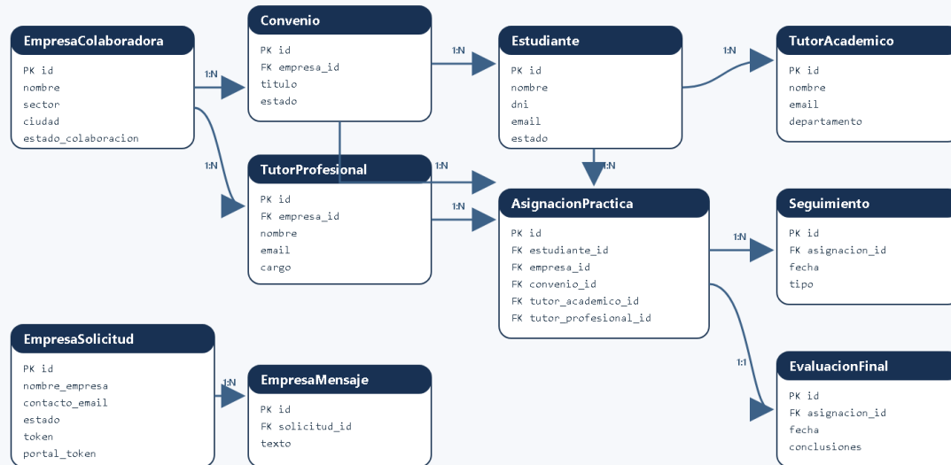
Esquema relacional simplificado de la base de datos
