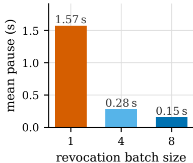
(b) amortisation
