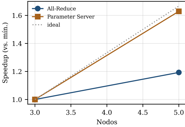
Figura 6: Speedup de throughput de 3 a 5 nodos (referencia: la propia config de 3 nodos). PS escala con mayor pendiente que AR desde una base más baja.
