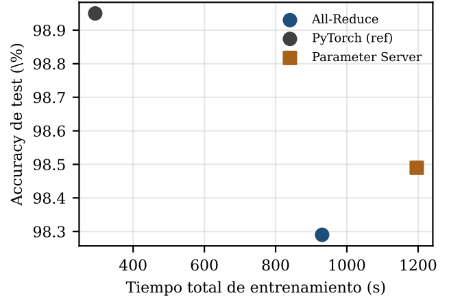
Figura 4: Accuracy de test vs. tiempo total (MNIST, nielsen, runs de referencia). All-Reduce alcanza \sim 98,3 % antes que Parameter Server; el baseline single-process es el más rápido al no pagar comunicación.
