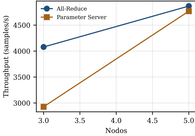
Figura 5: Throughput (samples/s) vs. nodos, batch por worker fijo. AR domina pero PS recorta distancia al crecer los nodos.
