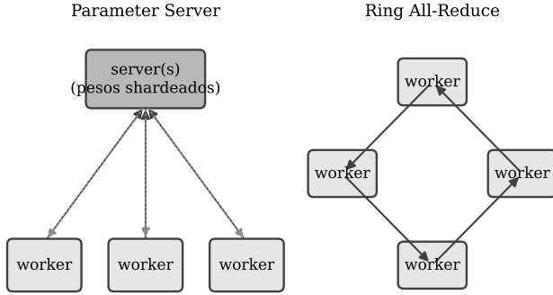
Figura 2: Parameter Server (izquierda): los workers hacen push/pull contra servidores centrales que pueden shardear los pesos. Ring All-Reduce (derecha): los workers promedian gradientes entre sí sin servidor central.
