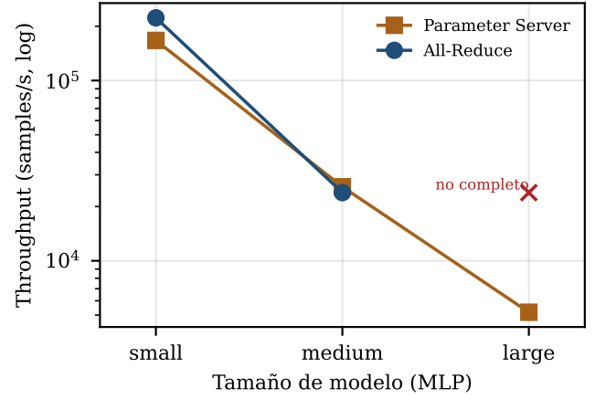
Figura 7: Presión de comunicación: throughput (log) vs. tamaño de MLP a 3 nodos. La ventaja de AR en modelos pequeños se diluye al crecer el gradiente; con el modelo grande AR no completó el entrenamiento (marca roja) y PS sí.
