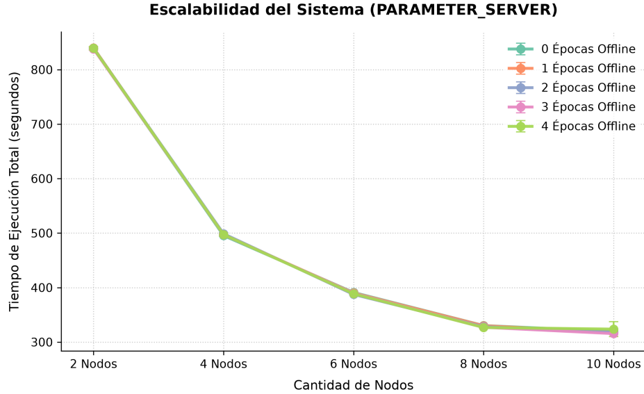
Figura 7: Comparación de tiempos de ejecución bajo distintas cantidades de épocas offline con Parameter Server.
