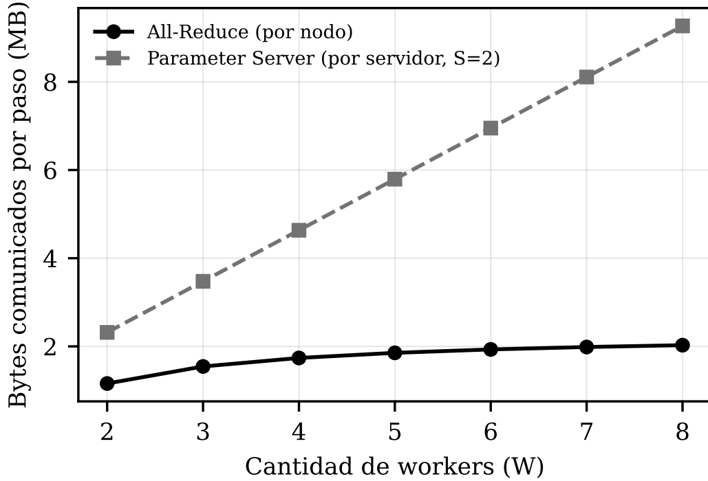
Figura 5: Volumen de datos comunicado por paso (métrica analítica, independiente de la red) frente al número de workers. En All-Reduce el volumen por nodo es casi constante; en Parameter Server el tráfico por servidor crece con los workers.
