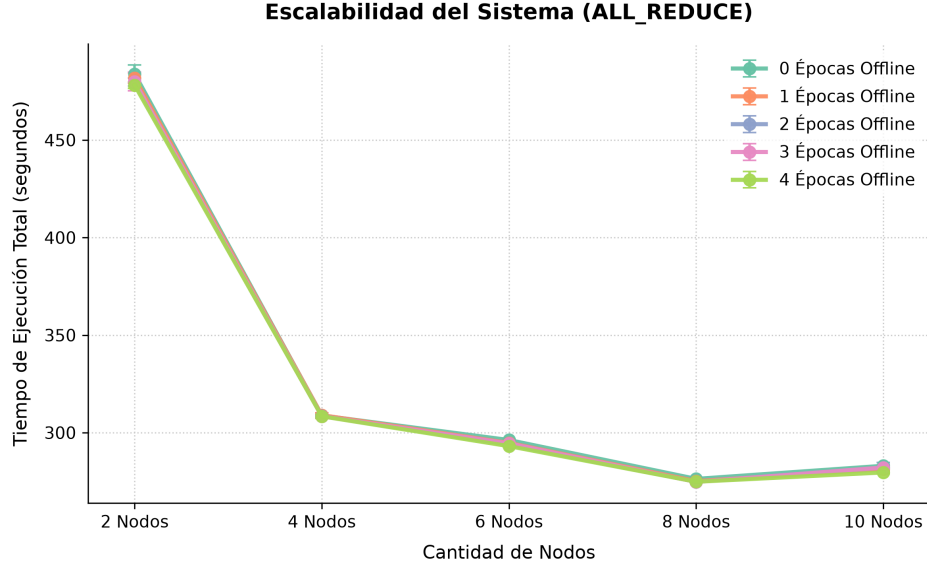
Figura 6: Comparación de tiempos de ejecución bajo distintas cantidades de épocas offline con All-Reduce.
