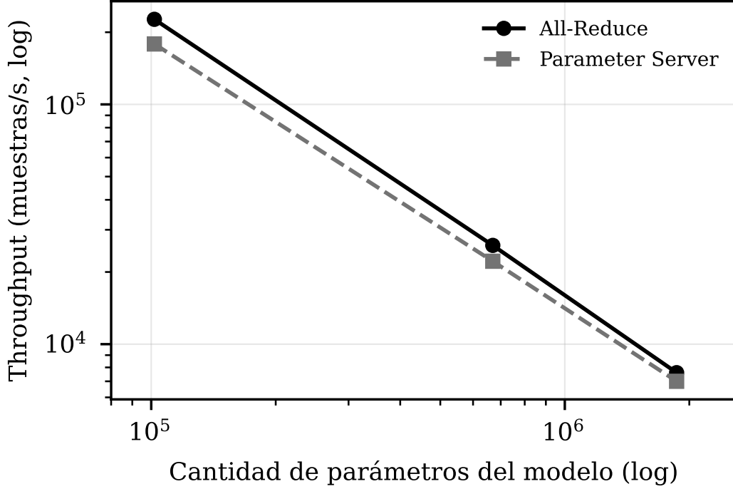
Figura 4: Presión de comunicación: throughput (escala logarítmica) frente al tamaño del modelo (escala logarítmica) a 3 workers. All-Reduce sostiene mayor throughput en los tres tamaños; la ventaja se reduce al crecer el modelo.
