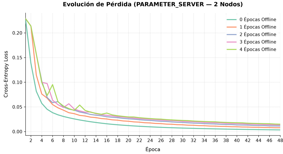
Figura 10: Trayectoria de pérdida con entropía cruzada exhibiendo ruido estocástico por cómputo offline en Parameter Server (2 nodos).
