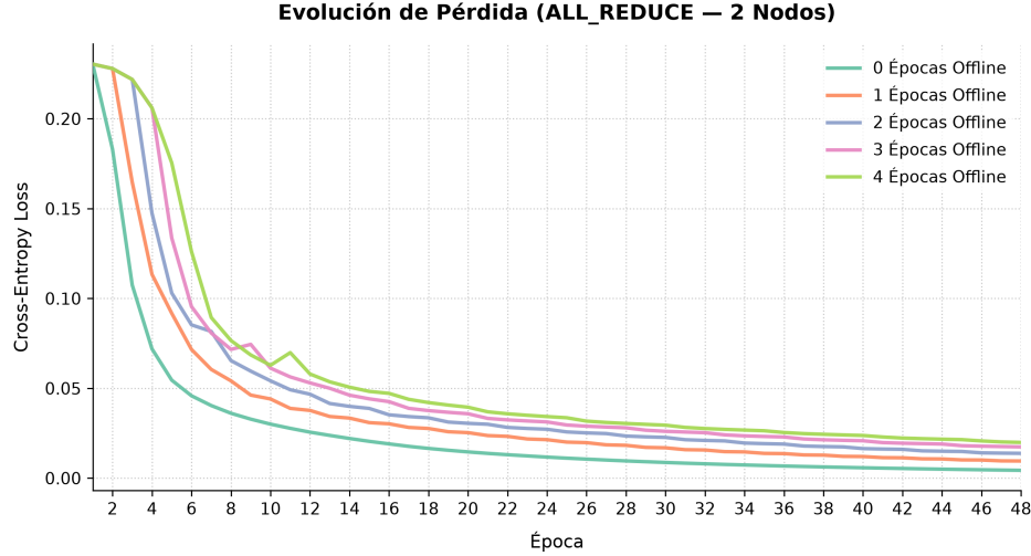
Figura 11: Trayectoria de pérdida con entropía cruzada exhibiendo ruido estocástico por cómputo offline en All-Reduce (2 nodos).
